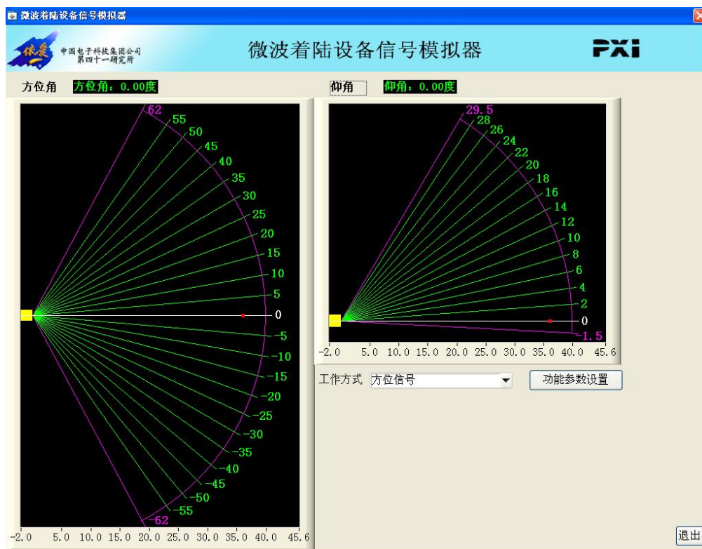
仪器面板主界面
