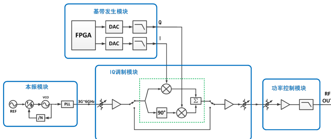
微波着陆设备信号模拟器原理框图
