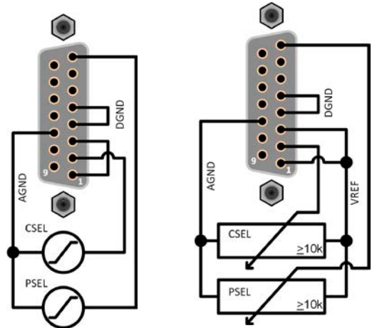
接电位器的范例
