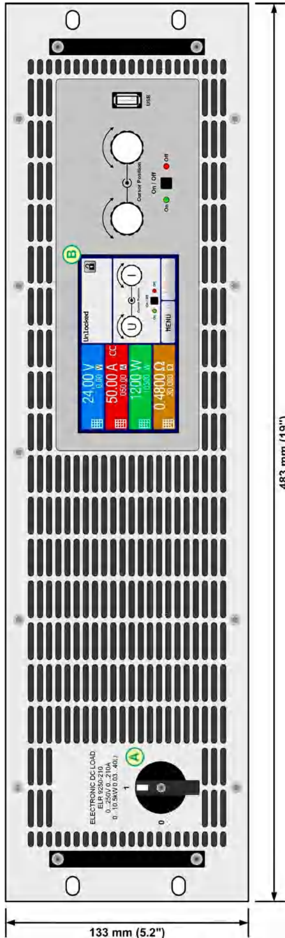
图 1 - 前视图
