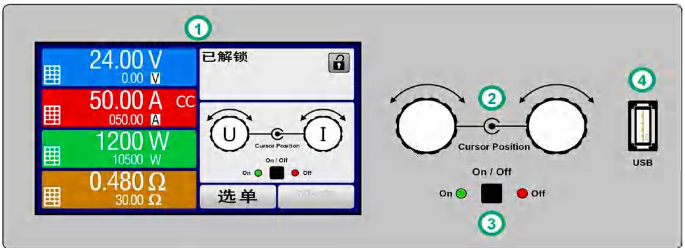
图 6 - 控制面板
