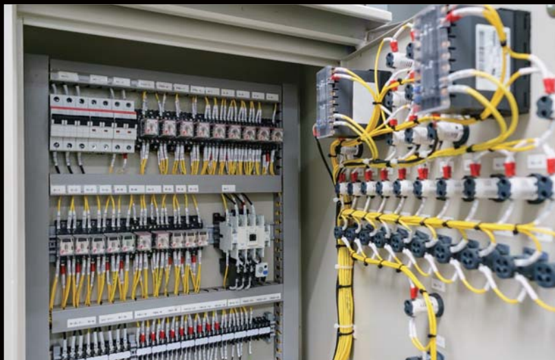
配电柜检测
