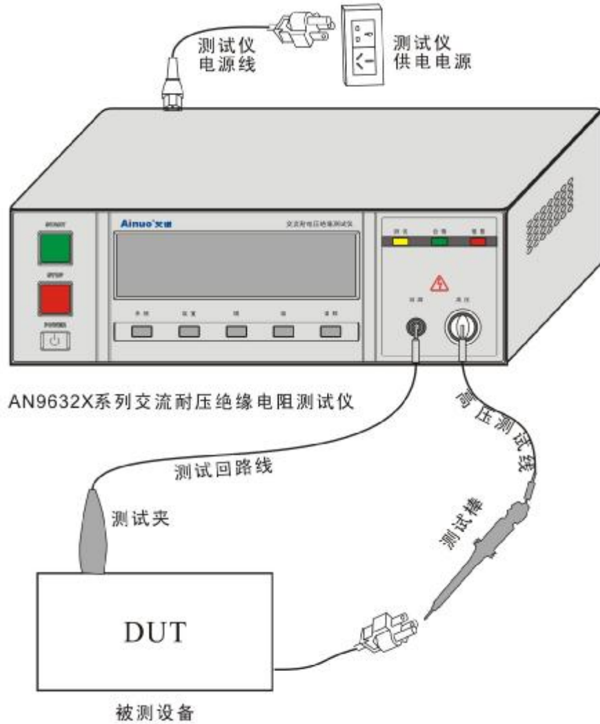
图 3.8.1 外部接线
