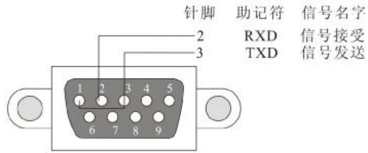
图 5.2.1 RS-232 接口
