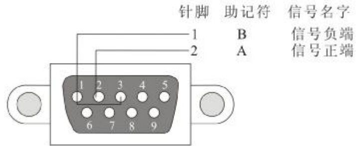
图 5.2.2 RS-485 接口
