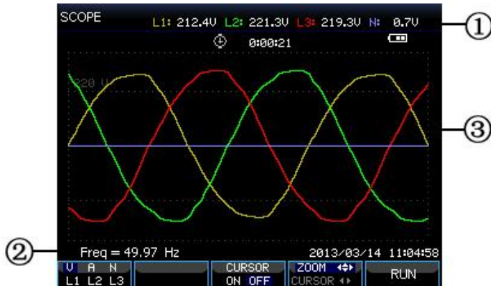
图 1-5-3 波形屏幕
