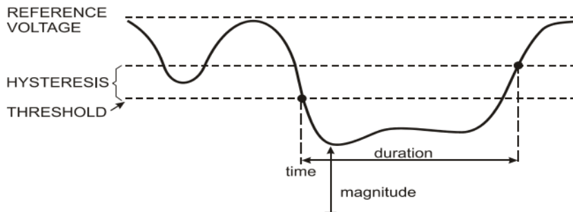
图 3-3-1 电压骤降的特征
