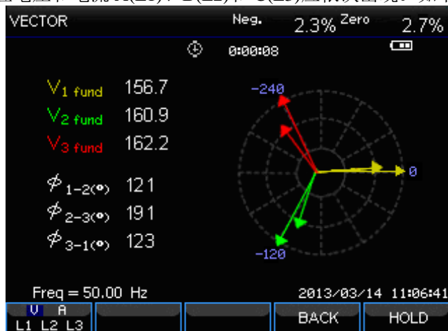
图 2-5-1 正确连接的分析仪矢量图
