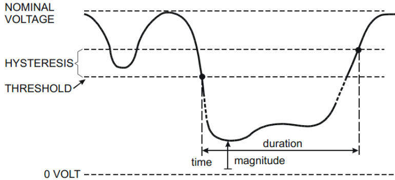
图 3-3-3 电压中断的特征
