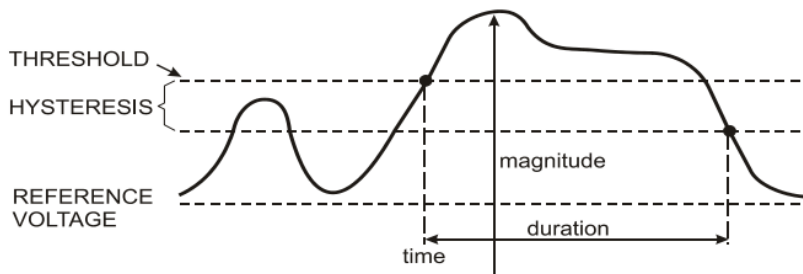
图 3-3-2 电压骤升的特征
