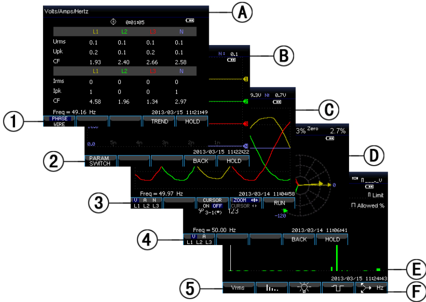
图 2-6-1 显示类型概览
