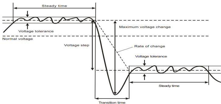
图 3-3-4 快速电压变化的特征
