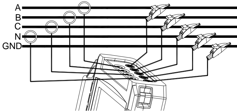
图 1-3-1 分析仪与三相配电系统连接
