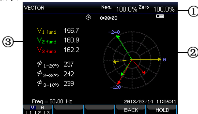
图 1-5-4 向量图屏幕
