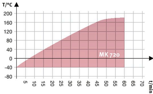
加热曲线图
