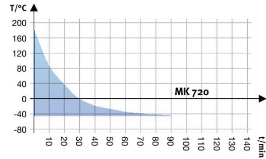
冷却曲线图
