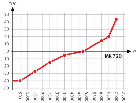
加热曲线图
