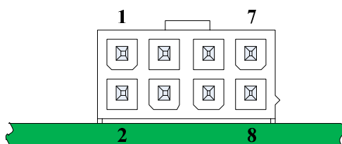
图 2:2 8PIN ATX8 测量接口示意图
