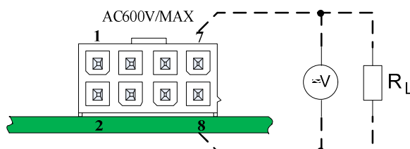
图 4:1 N8050A 通道 1 与外部电路接线示意图
