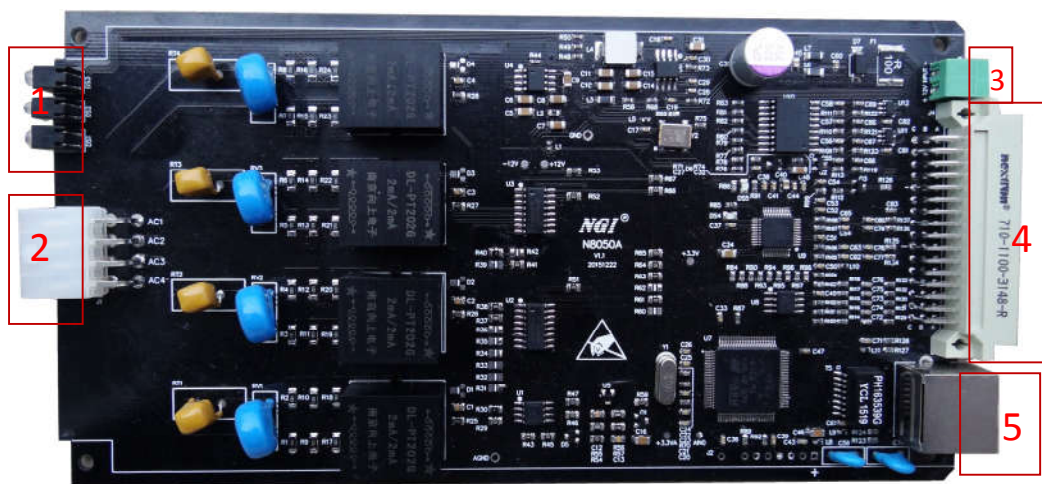
图 2:1 N8050A 实物图
