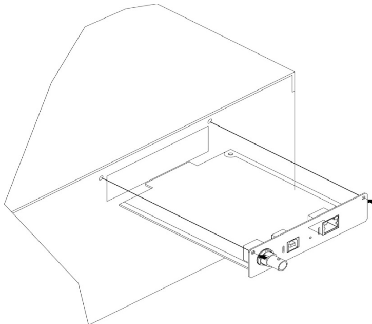
圖 2-5 選購卡(含 USB 及 Ethernet)
