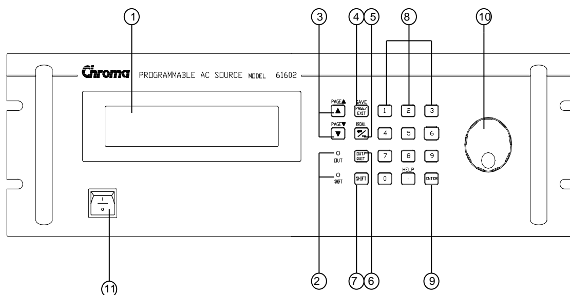
圖 1-1 前面板
