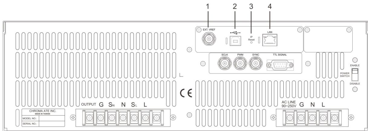
圖 2-3 後面板(含 USB 及 Ethernet)
