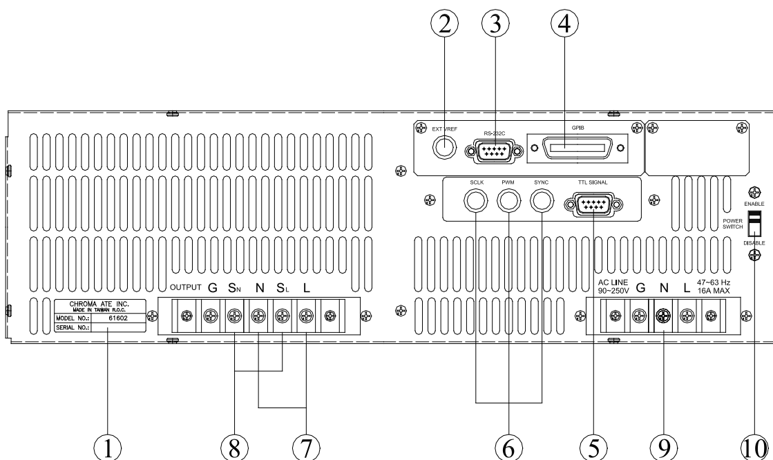
圖 1-2 後面板
