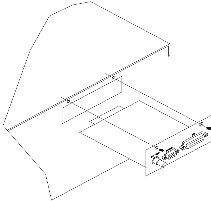
圖 2-4 選購板
