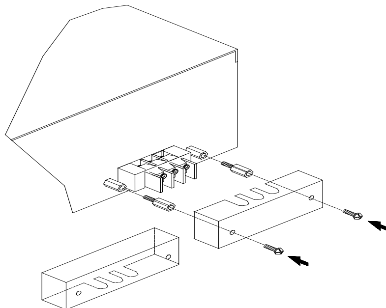
圖 2-2 輸入端子外殼
