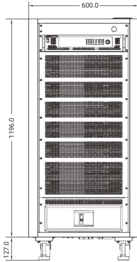
27U直流电源系统，单位：mm
