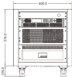
13U直流电源系统，单位：mm
