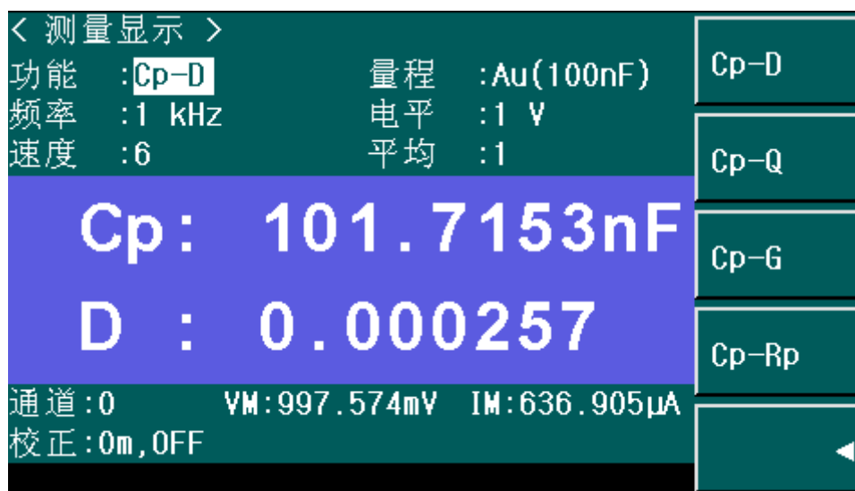
图 3-4 副参数选择菜单窗口
