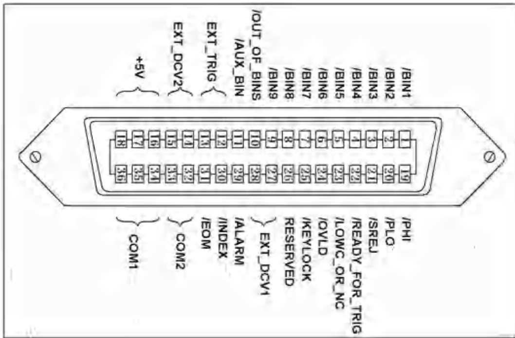
图 8-2 HANDLER 接口信号线定义
