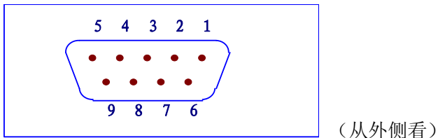
图 5-1 串行口连接器
