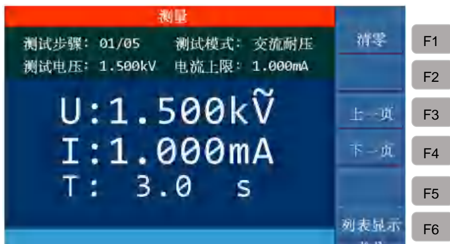
图 4-17.1 交流测量界面
