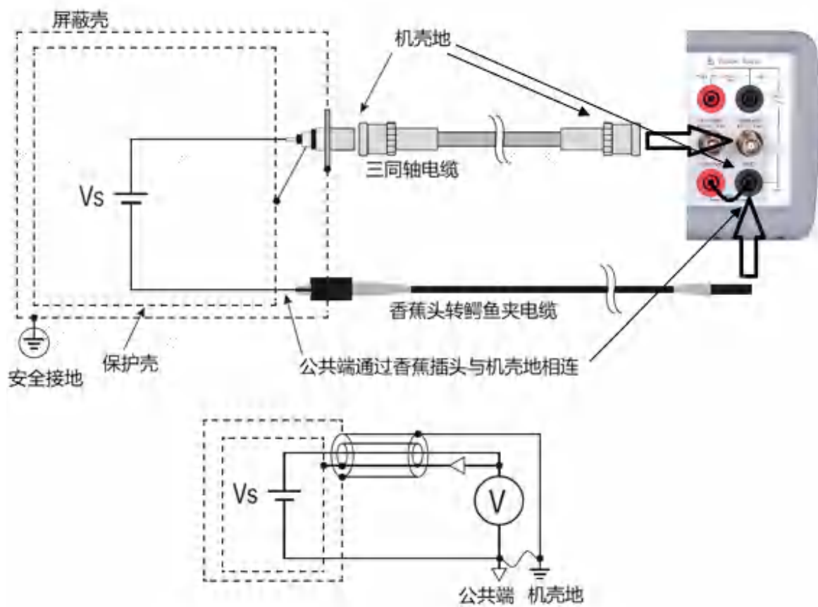
图 5-7 无保护的电压测量连接方式
