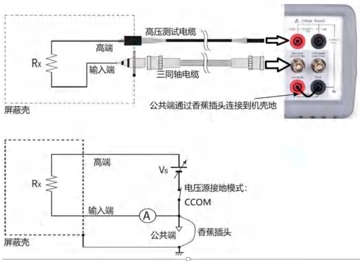
图 5-10 浮动设备的测量
