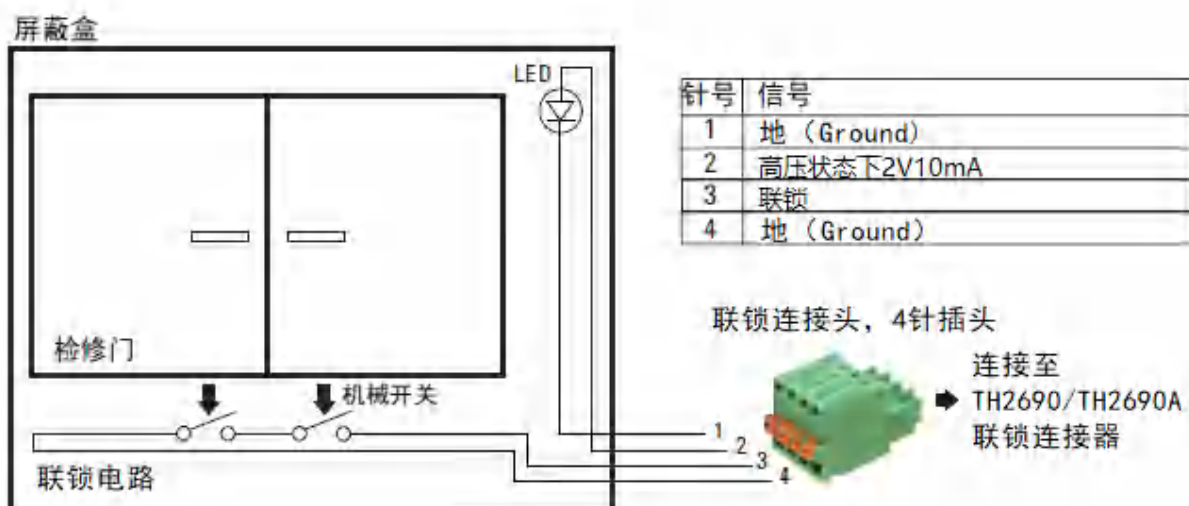
图 5-14 联锁电路
