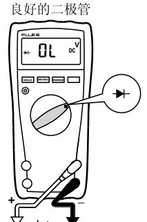
反向偏压
