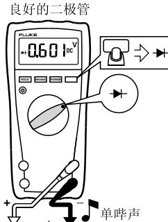
正向偏压
