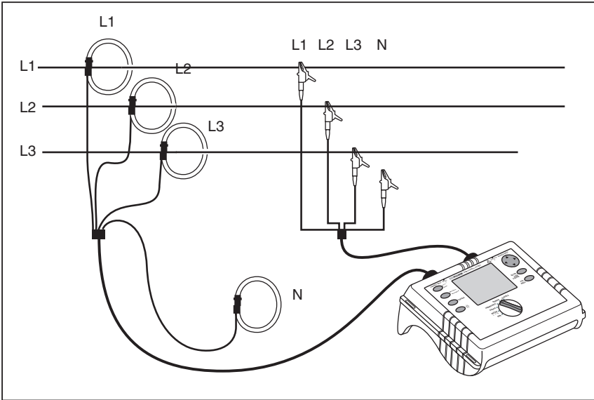
图 10. 三相三角形 \Delta 连接-Blondel (Aron, 二元三角形) 连接-Blondel" \f f
