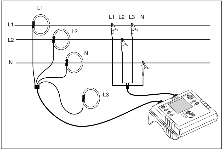
图 7. 分相连接
