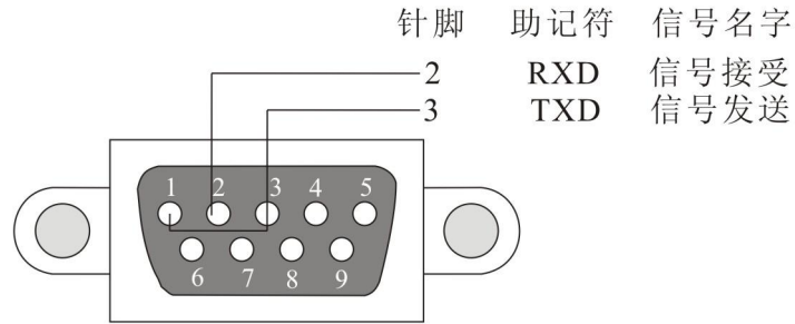
图 5.2.2 RS-485 接口
