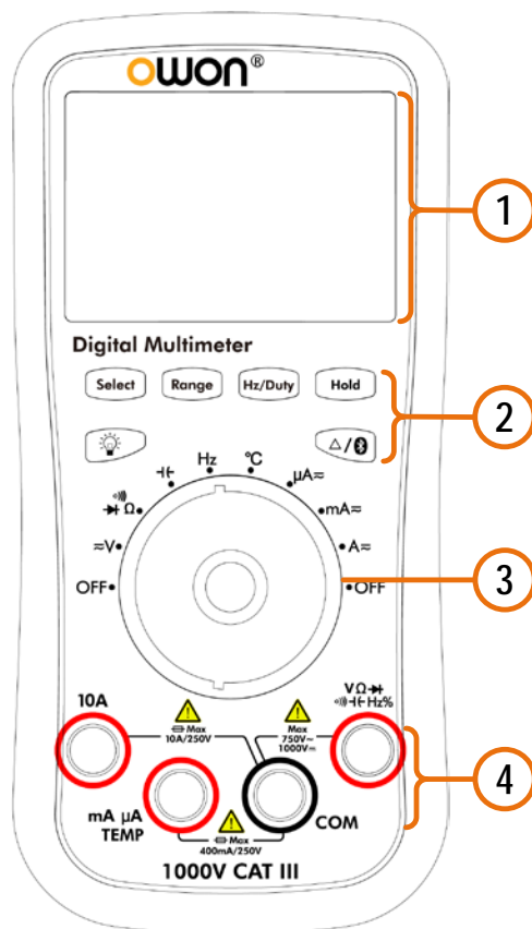
图 2-1 前面板概览
