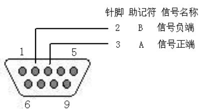
(1) RS-485 通讯口
