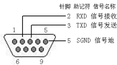
(2) RS-232 通讯口
