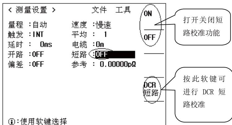
图 5-3 短路校正功能
