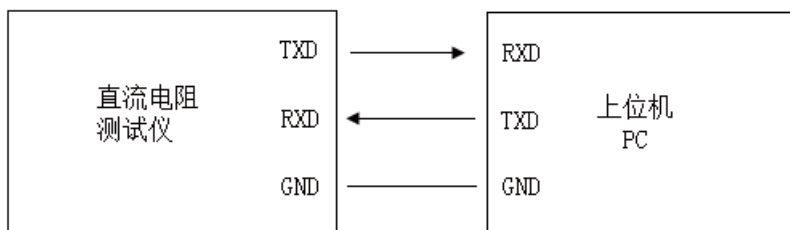
图 7-1 PC 与直流电阻测试仪连接图
