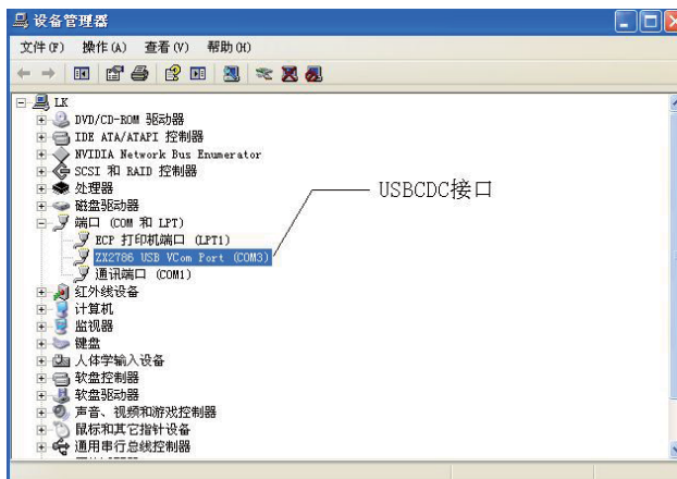
图 7-7 设备管理器显示仪器 USB VCom Port
