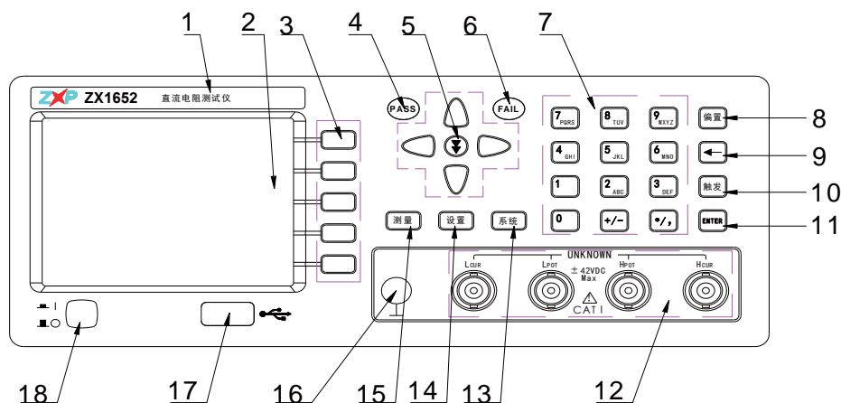
图 2-1 直流电阻测试仪前面板
