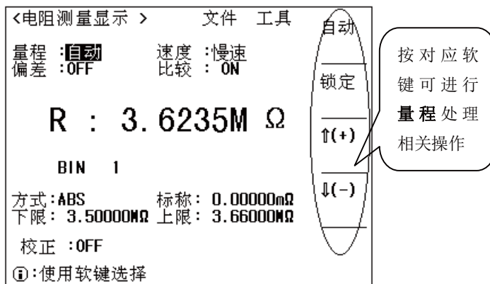
图 4-4 量程操作设置界面
