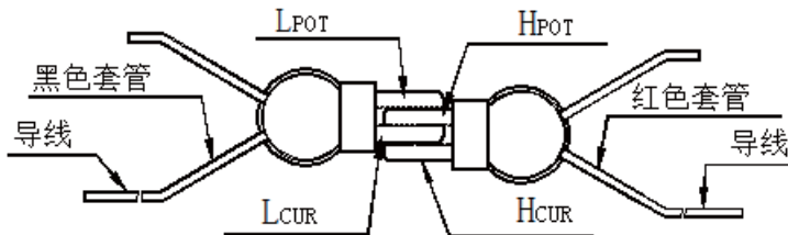
图 9-1 短路清零测试夹连接图
