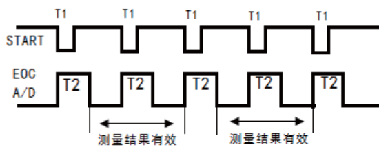
图 8-5 仪器工作时序图
