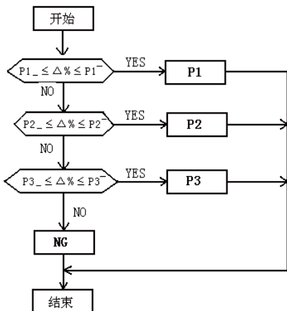
图 8-2 3 BIN 分选流程图
