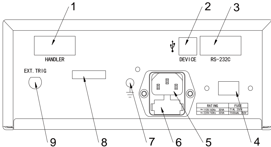
图 2-2 直流电阻测试仪后面板
