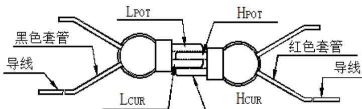
图 5-4 测试夹短路正常连接图
