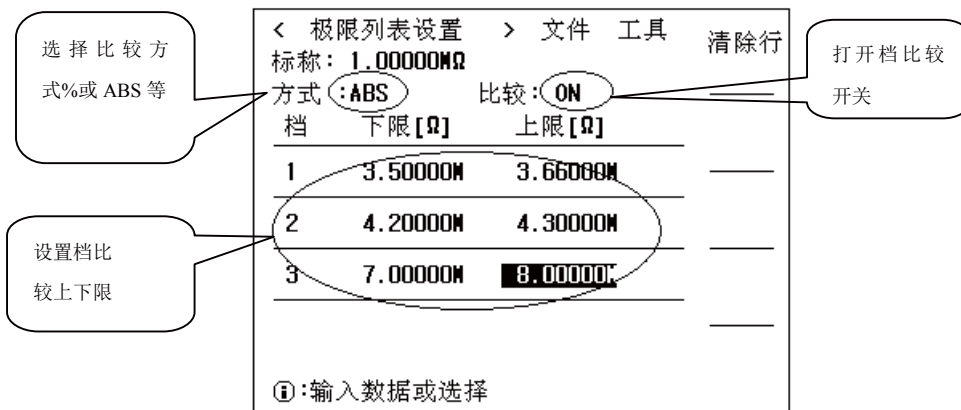
图 4-7<极限列表设置>四档设置页面
