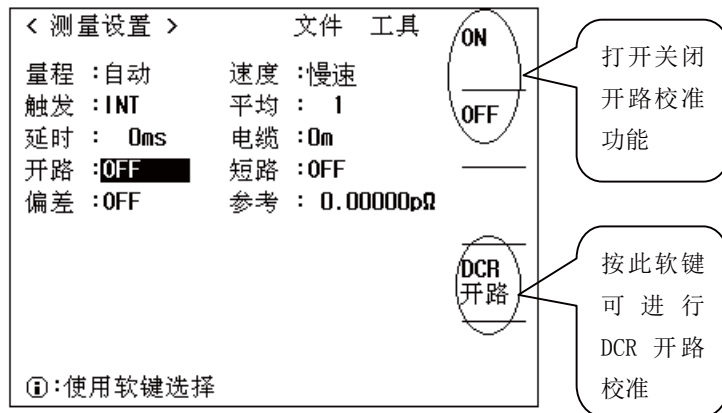
图 5-2 开路校正功能
