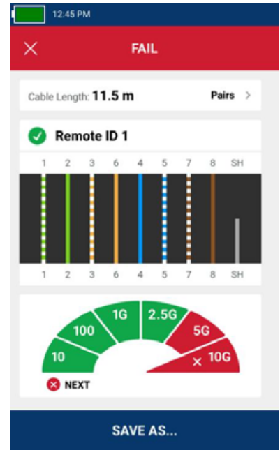
连接了远端单元的线缆测试 显示远端 ID 高达 1 Gb/s，但由于用户设 置的性能限值为 10 Gb/s 而未能通过测试。
