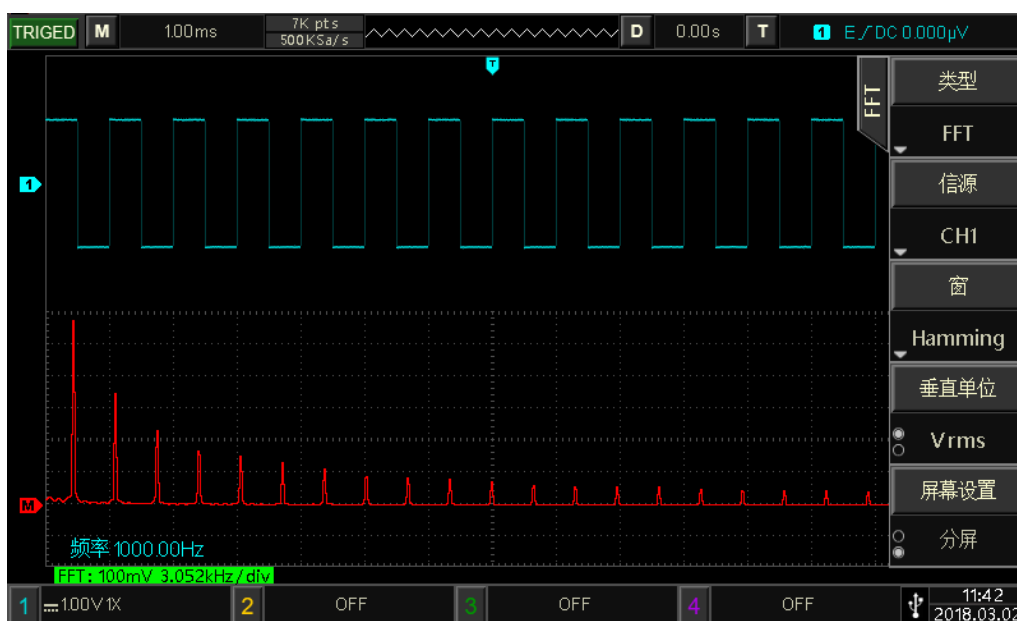
图 5-1 FFT 频谱
