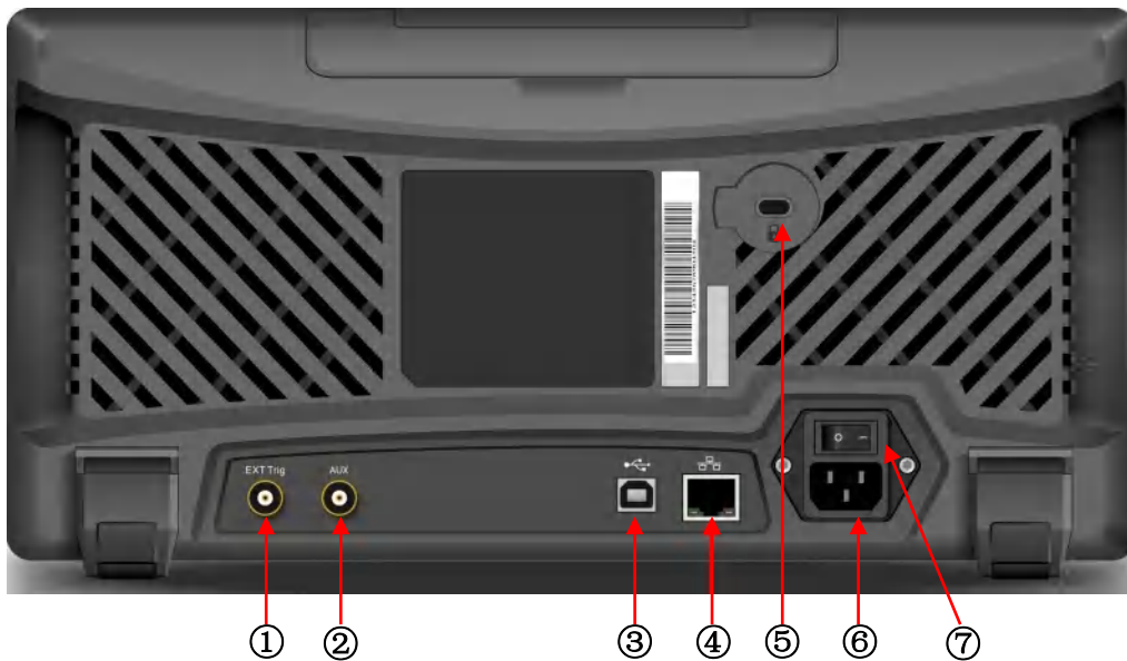
图 1-4 示波器后面板
