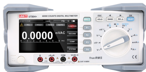
■ UT804+
