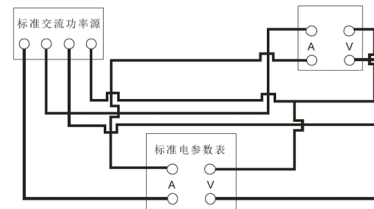
图19 检定和校准接线图
