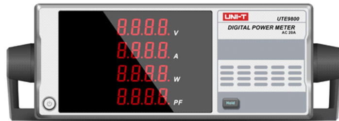
图5 UTE9800前面板
