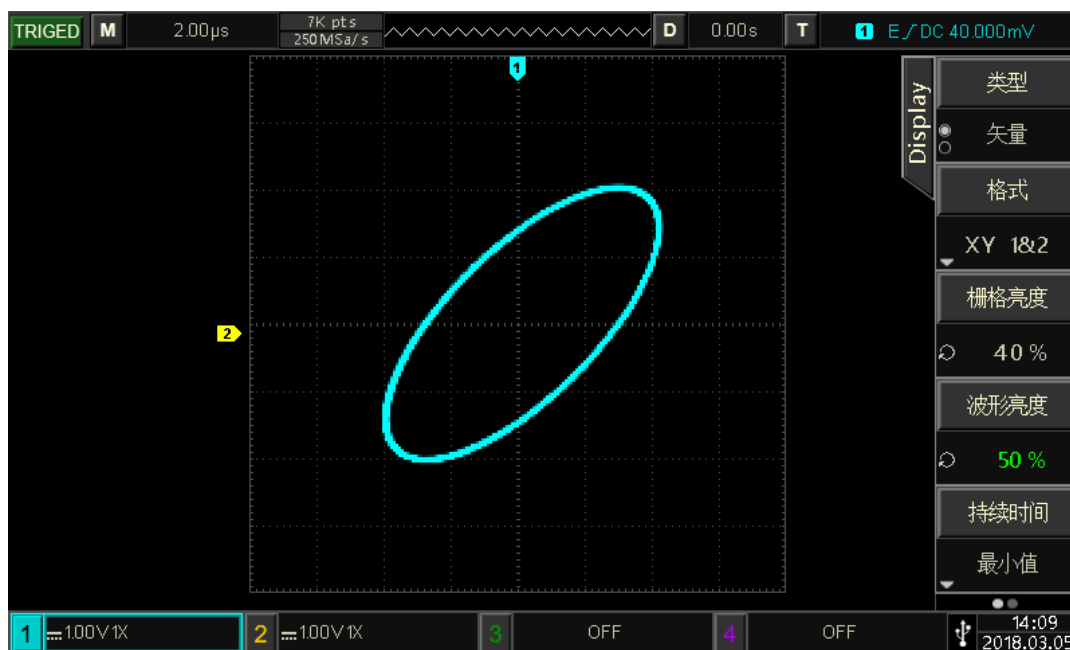
图 7-1 XY 模式下的波形显示
