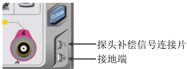
图 1-1 探头补偿信号连接片和接地端
