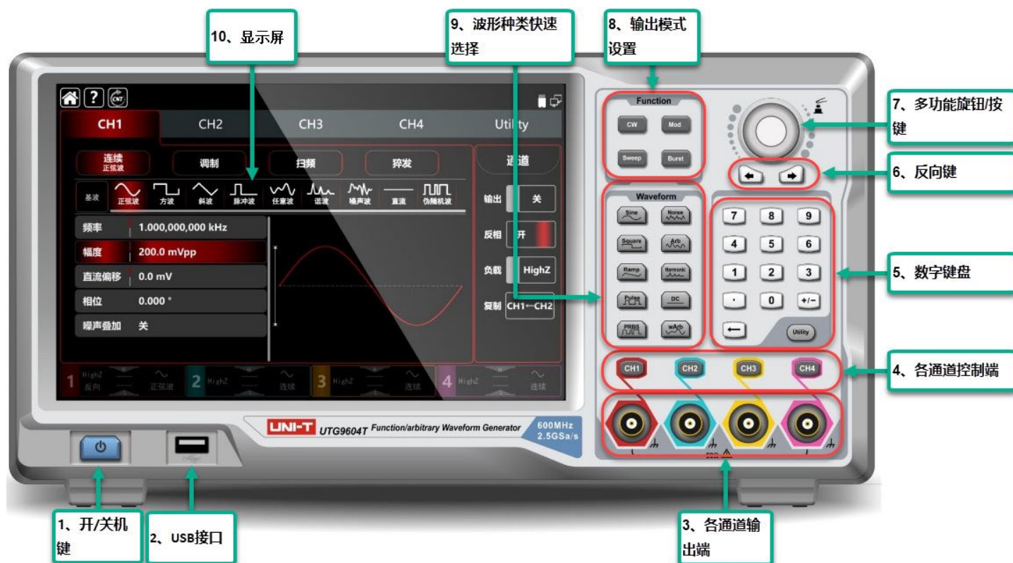
图 2-1 前面板结构图
