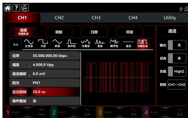
图 2-13 伪随机波设置
