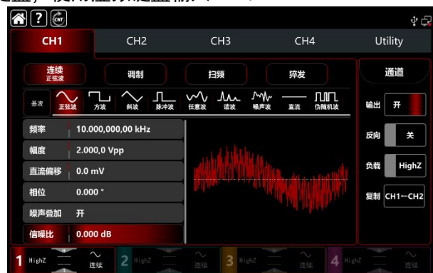
图 2-14 噪声叠加
