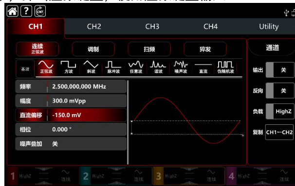
图2-6 直流偏移设置
