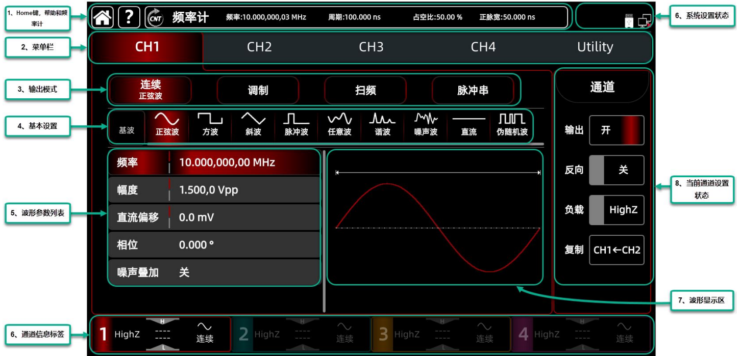
图2-3 触摸显示界面图
