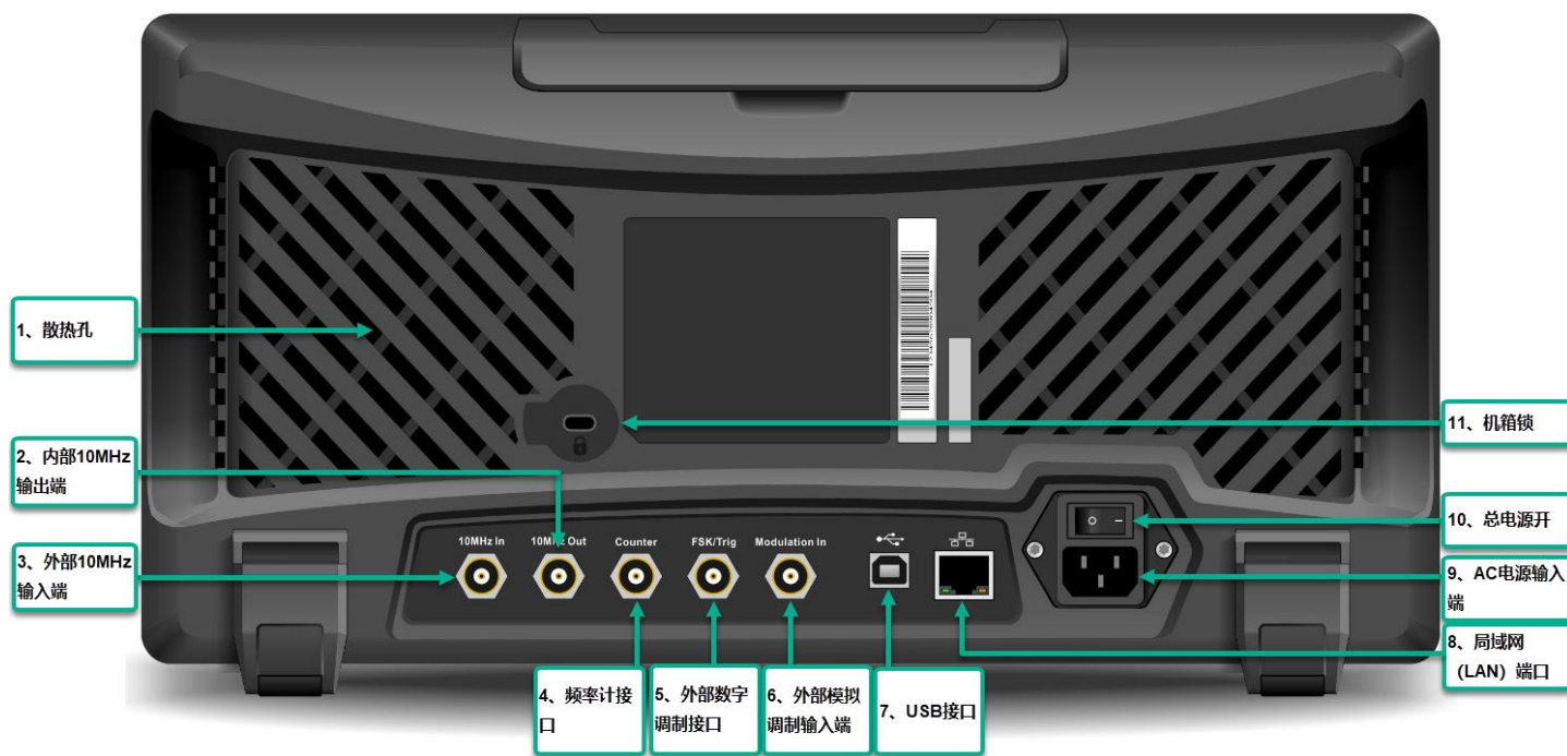
图 2-2 后面板结构图
