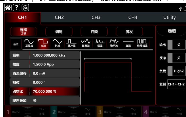
图2-7 方波设置
