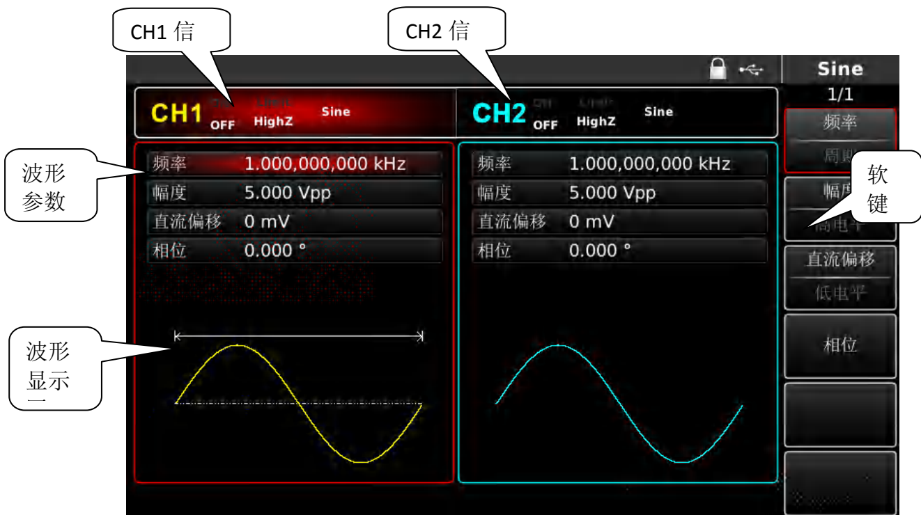
图 2-3 功能界面
