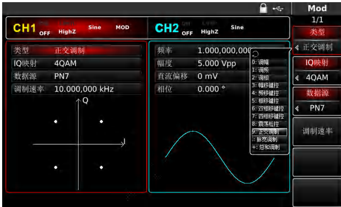
图 4-92 选中正交调制功能
