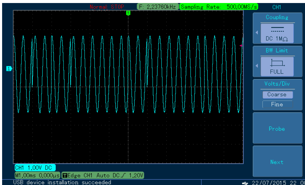
图 4-72 示波器观察双相移键控波形
