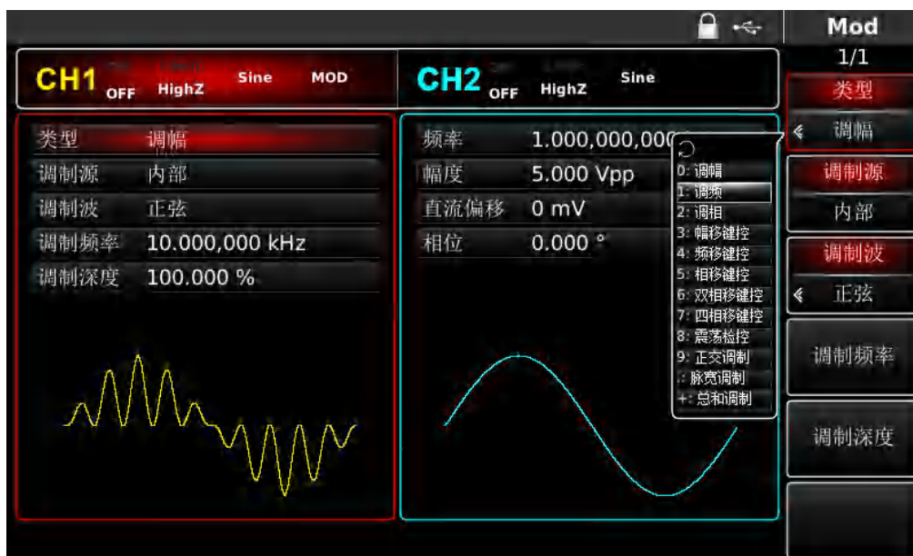
图 4-14 选中频率调制
