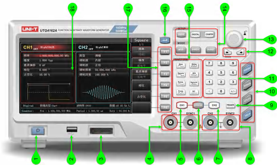
图 2-1 前面板结构图
