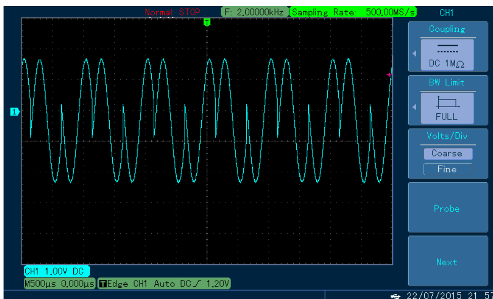
图 4-63 示波器观察相移键控波形
