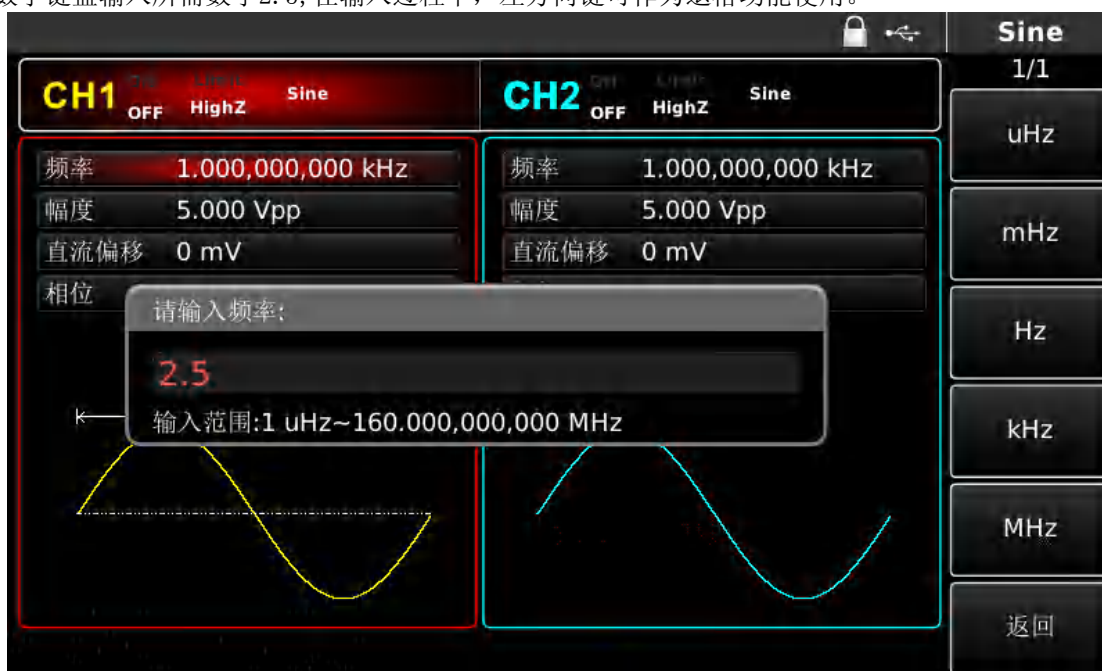
图 3-2 设置频率
