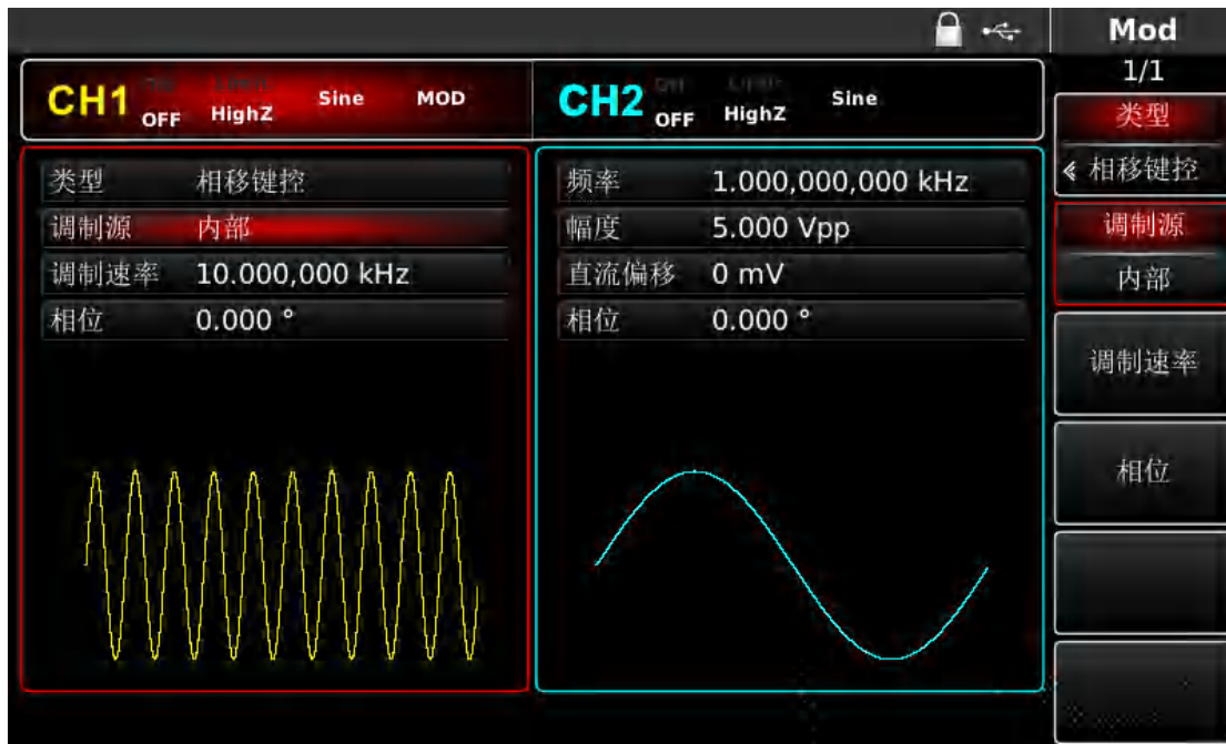
图 4-58 选择调制源
