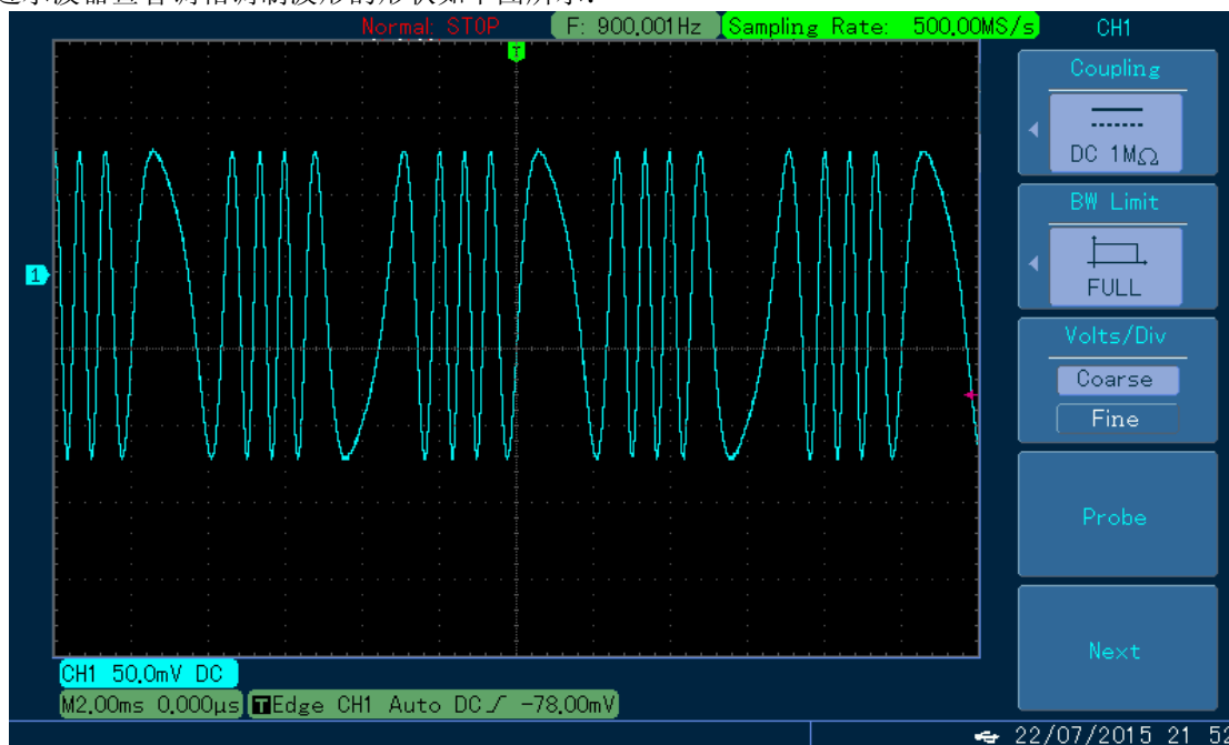
图 4-36 示波器观察调相波形
