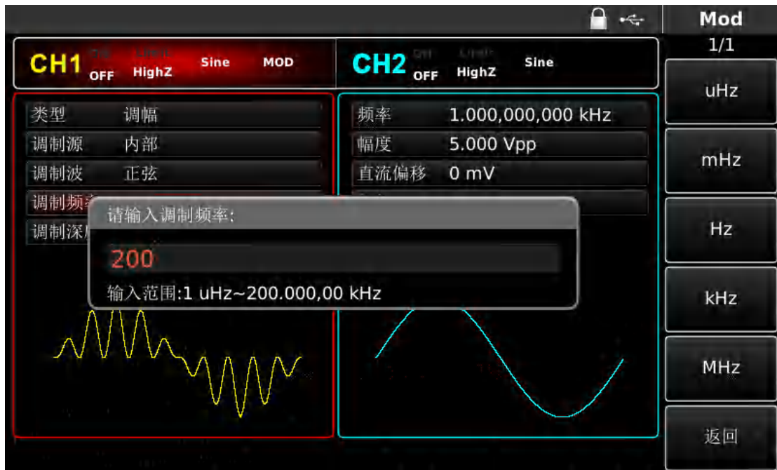
图 4-6 设置调制源频率
