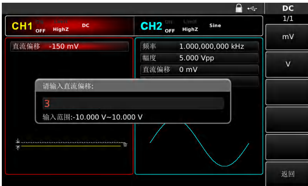
图3-7设置直流电压
