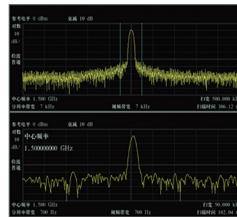
9 不同分辨率带宽显示效果,最小分辨率带宽达1Hz
