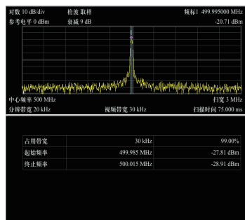
4 占用带宽测量
