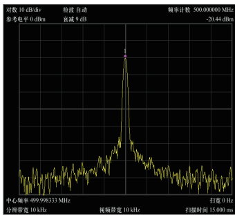
8 频率计数功能测量
