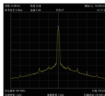
6 优异相噪指标
