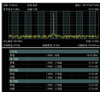
2 邻道功率测量
