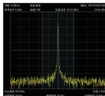
3 信道功率测量
