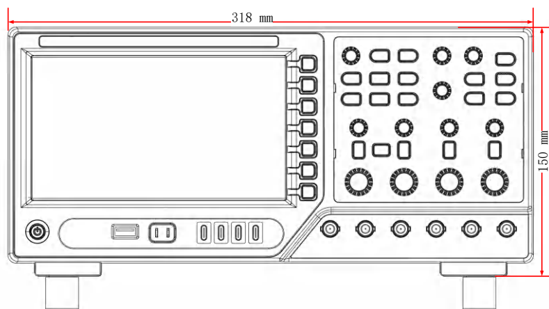
正视图
