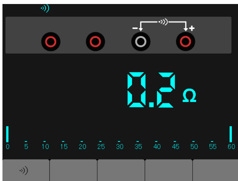
图4-4 通断测量
