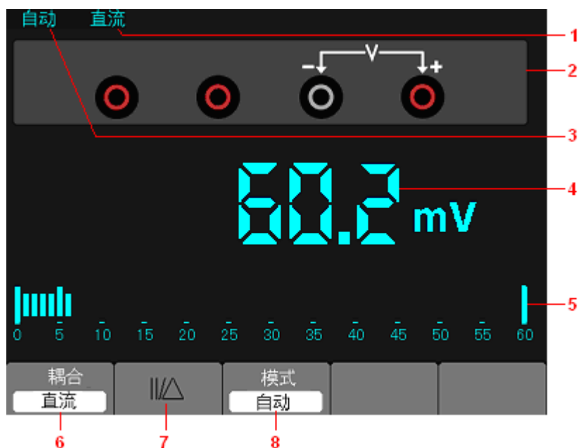
图4-1万用表界面
