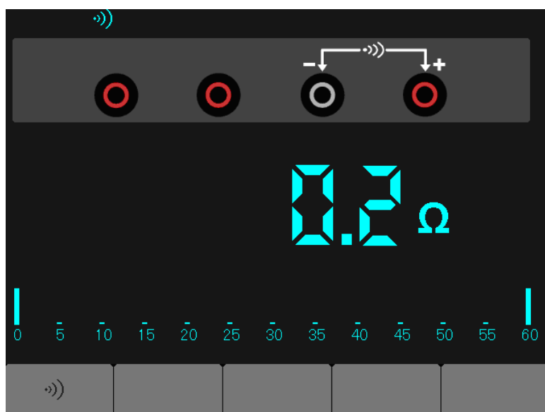
图4-4 通断测量
