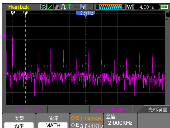
频率光标
