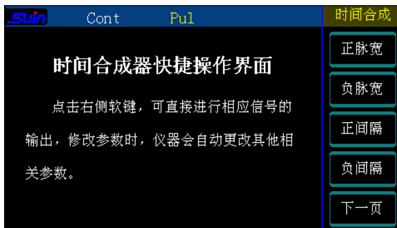
图 1-4 时间合成屏幕显示窗口
