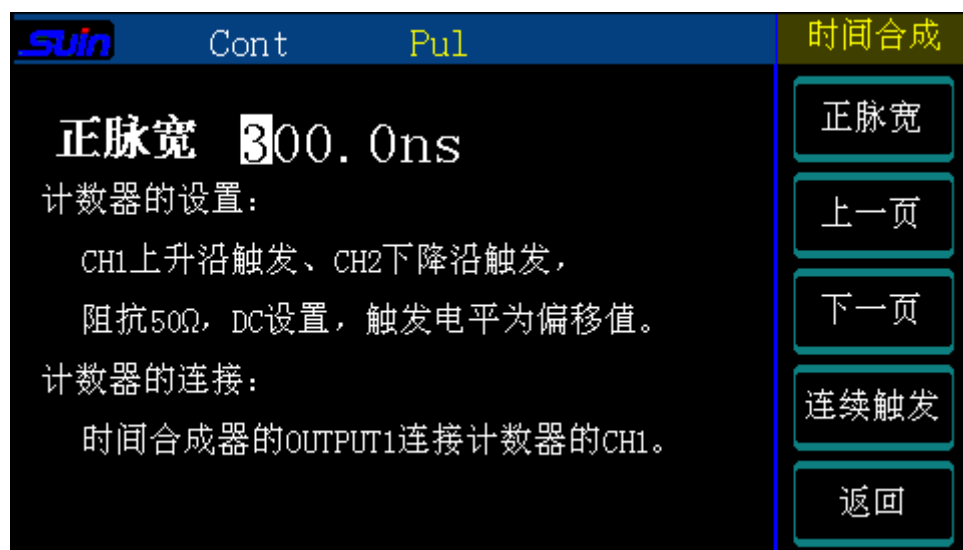
图 1-8 脉宽信号设置图
