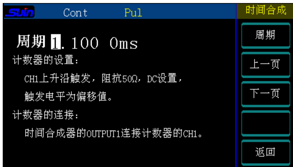
图 2-10 周期信号设置图
