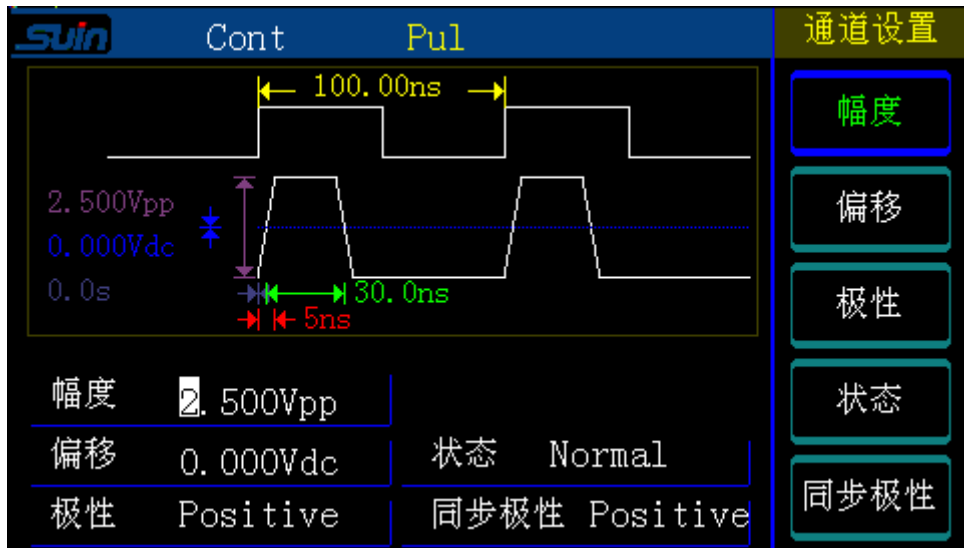
图 1-7 通道屏幕显示窗口
