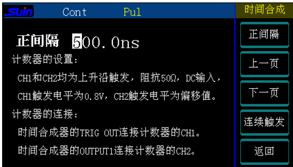
图 2-9 时间间隔设置图
