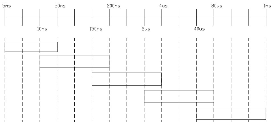
图 2-4 边沿时间约束范围
