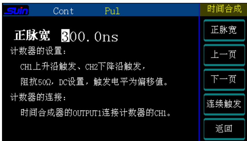
图 2-8 脉宽信号设置图
