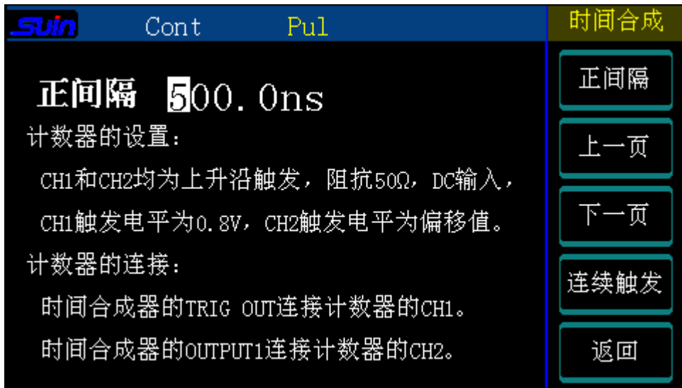
图 1-9 时间间隔信号设置图
