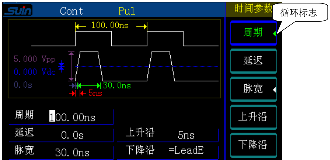
图 1-6 定时参数显示窗口
