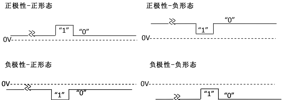
图 2-6 极性和状态转换分解图
