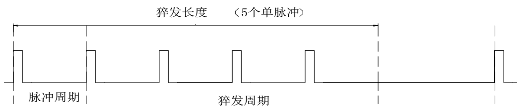
图 2-2 猝发波形示意图
