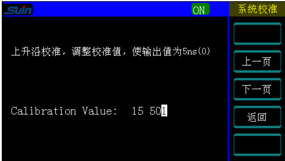
图 2-13 边沿校准屏幕
