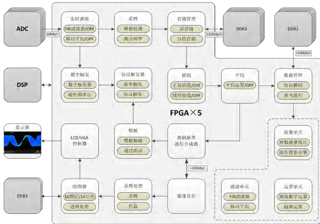
图 3.3 ZDS5000 系列示波器系统框图
