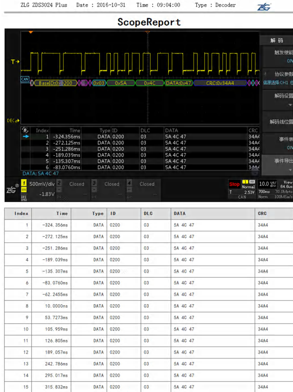
图 22.19 解码事件表报表实例
