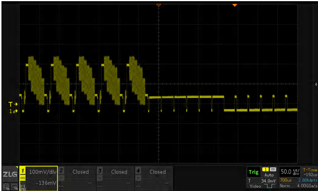
图 21.10 视频触发
