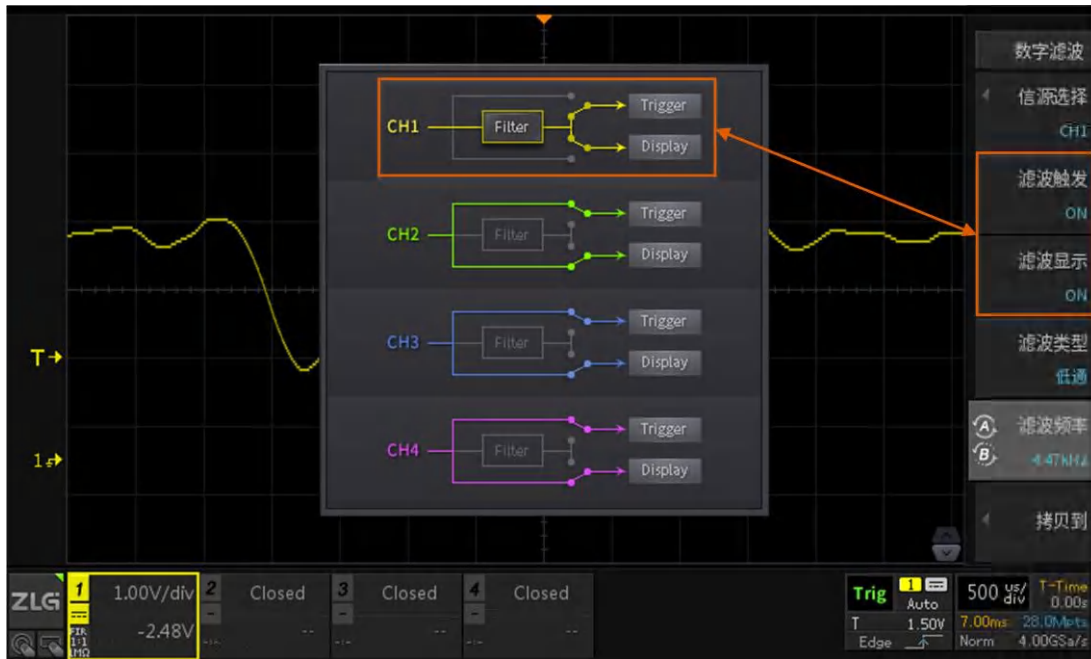
图 16.3 滤波触发和显示
