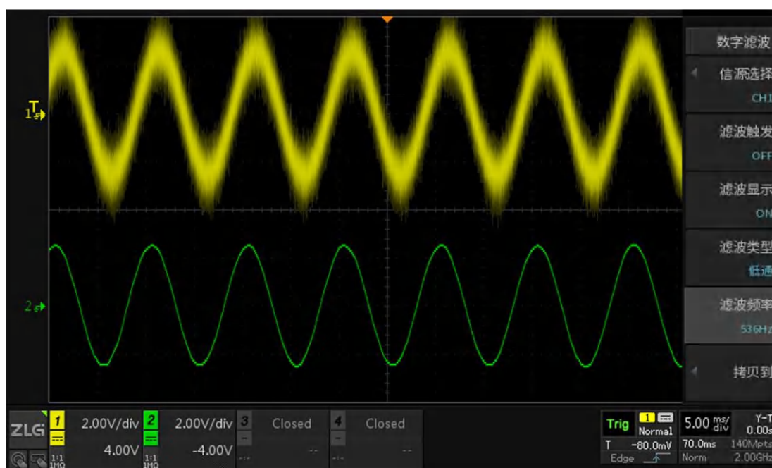
图 16.6 噪声滤波效果图
