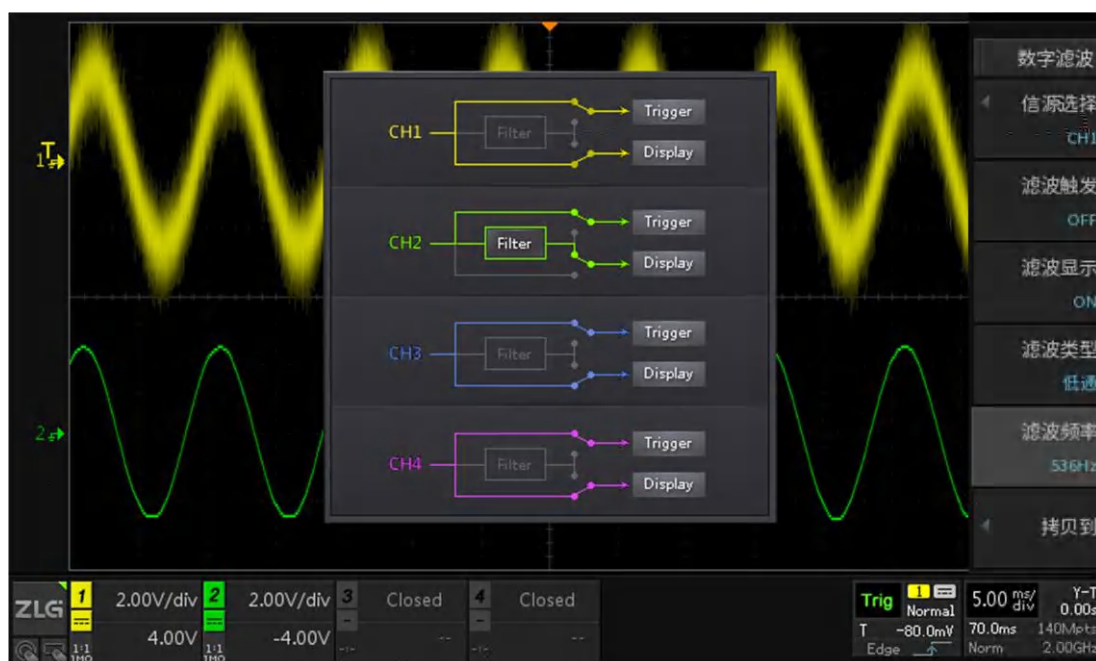
图 16.5 噪声滤波设置
