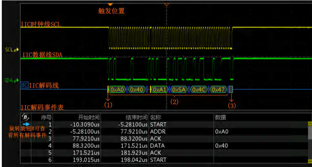
图 15.1 解码功能示意（ZDS5054Pro 型）
