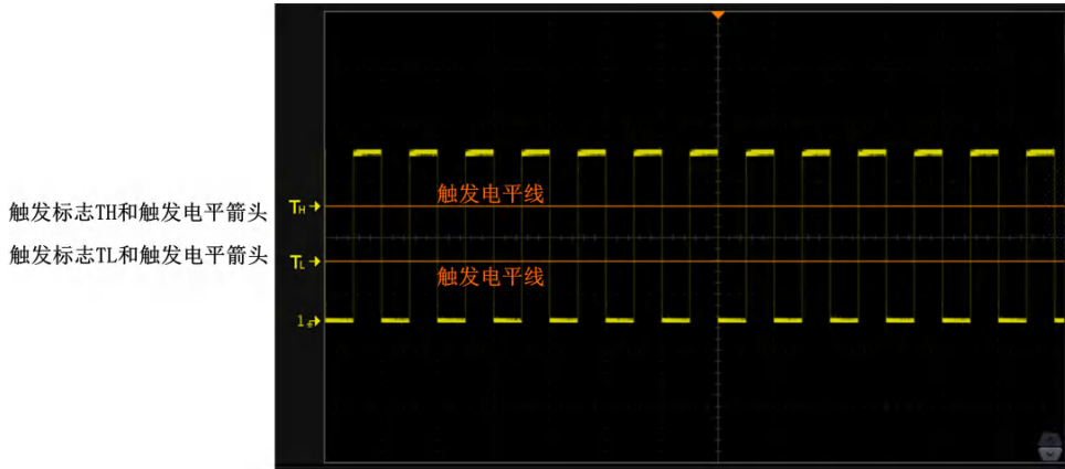
图 10.3 TH 和 TL 触发标志
