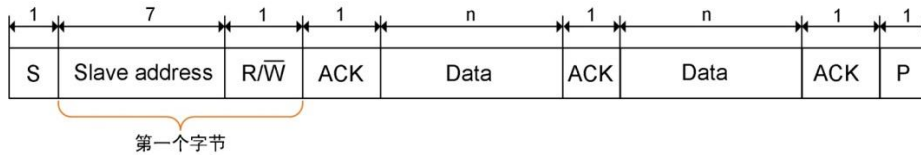
图 15.22 7 位寻址
