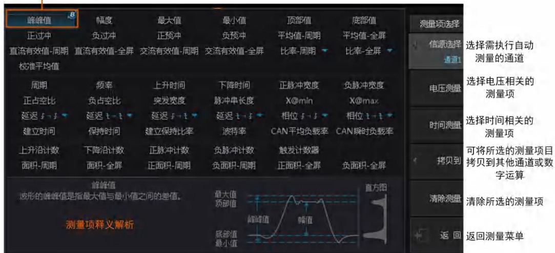
图 12.5 测量项设置
