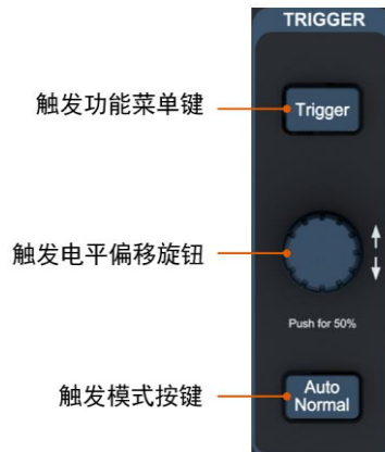
图 10.1 触发面板功能
