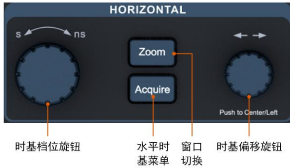
图 6.6 水平控制区
