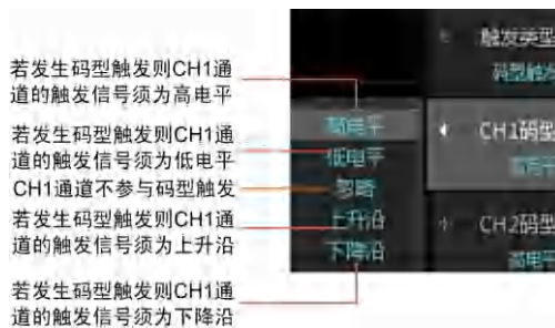
图 10.46 码型触发设置
