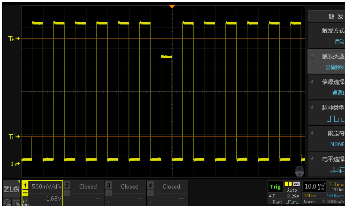
图 10.10 欠幅触发
