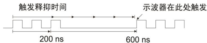
图 10.13 触发释抑时间设置
