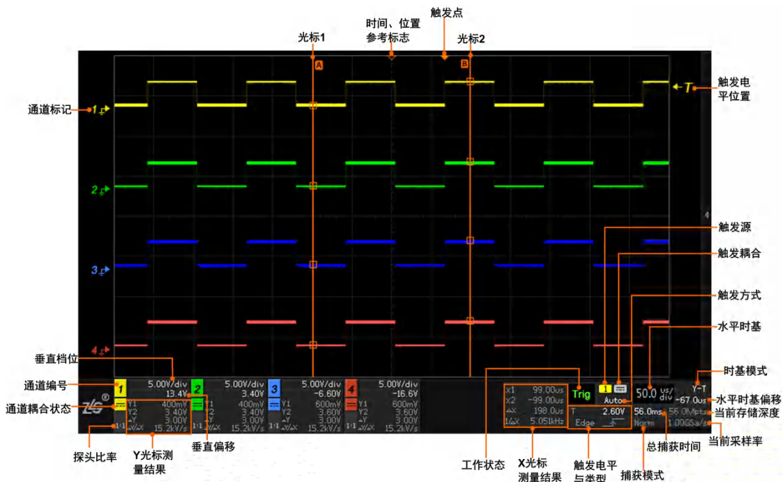
图 5.17 面板组件
