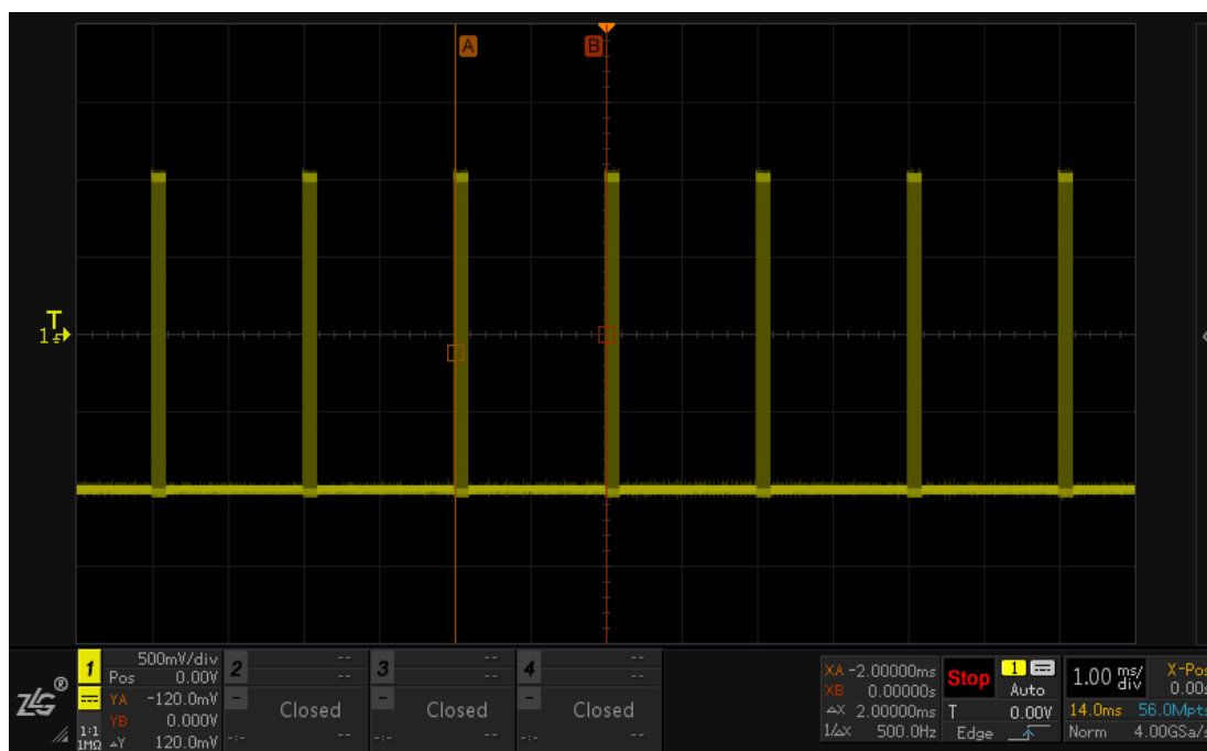
图 20.14 自定义波形显示
