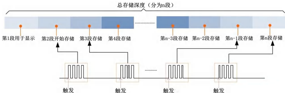
图 19.1 分段存储结构图
