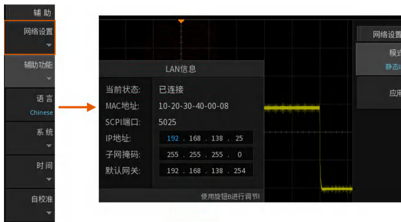
图 23.2 LAN 设置
