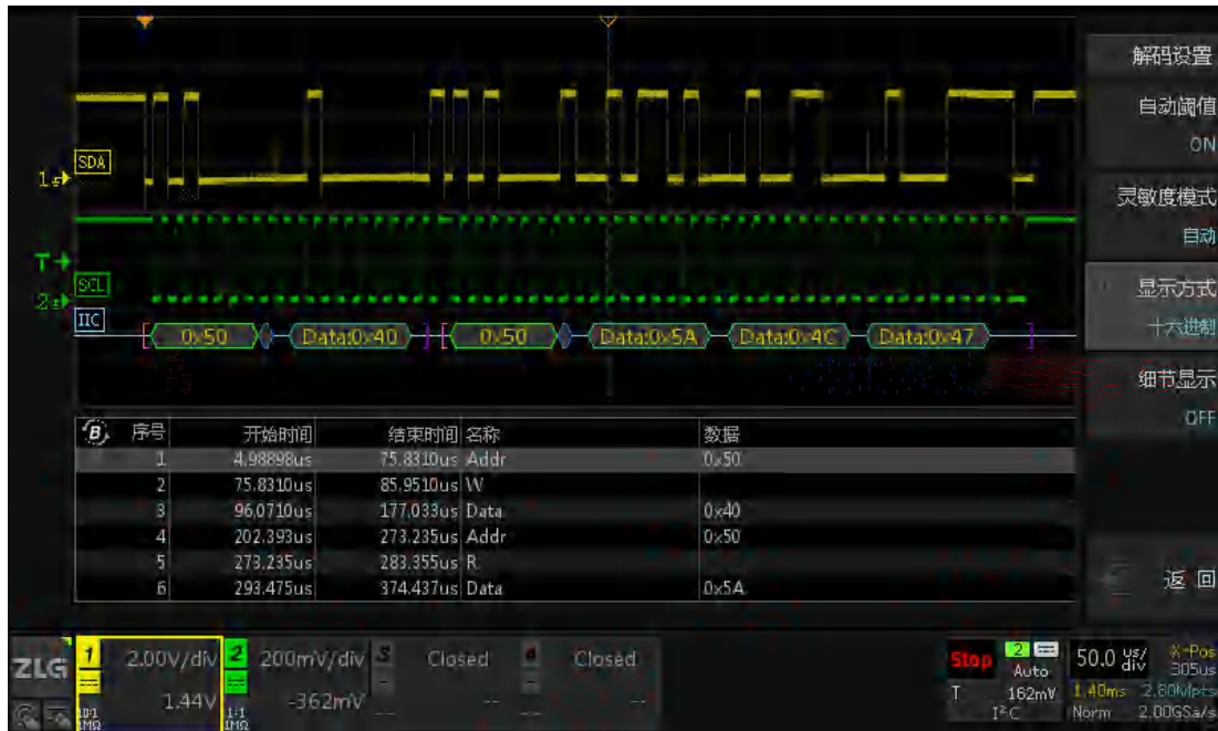
图 15.27 十六进制显示
