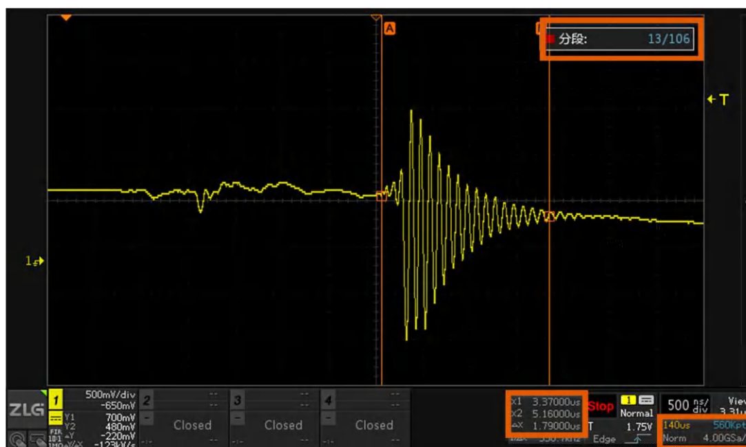
图 19.7 分段存储
