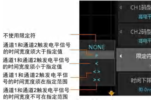
图 10.47 限定符设置说明
