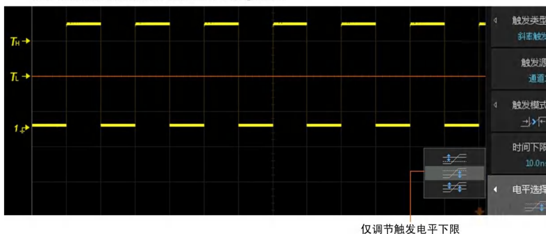
图 10.27 仅调节触发电平下限
