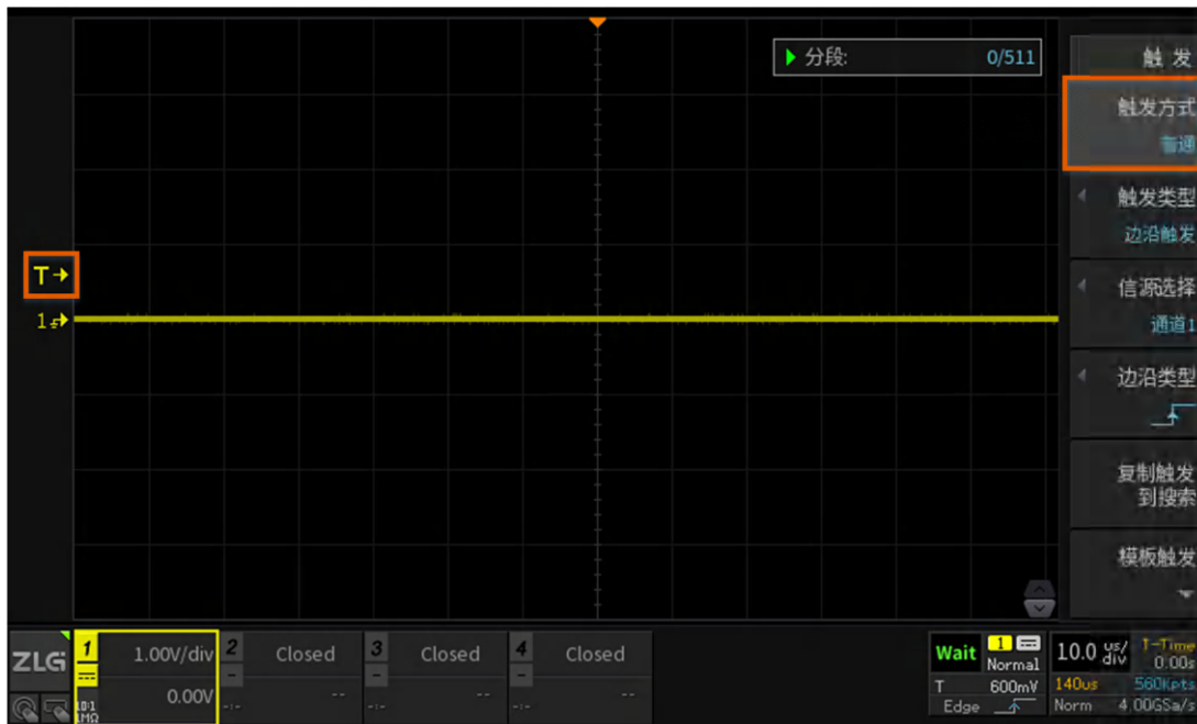
图 19.3 触发方式设置
