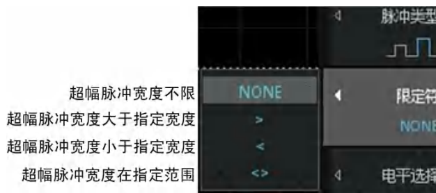
图 10.34 超幅触发的限定符
