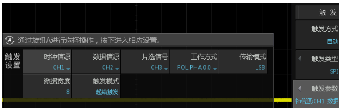
图 10.56 SPI 触发协议参数
