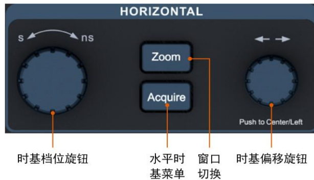
图 5.11 水平控制区
