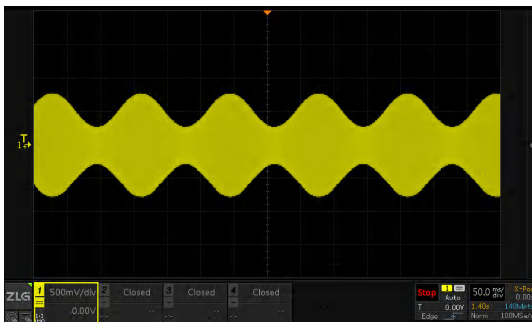
图 20.7 调制效果图
