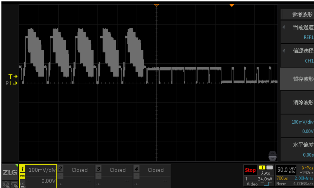
图 21.11 暂存波形
