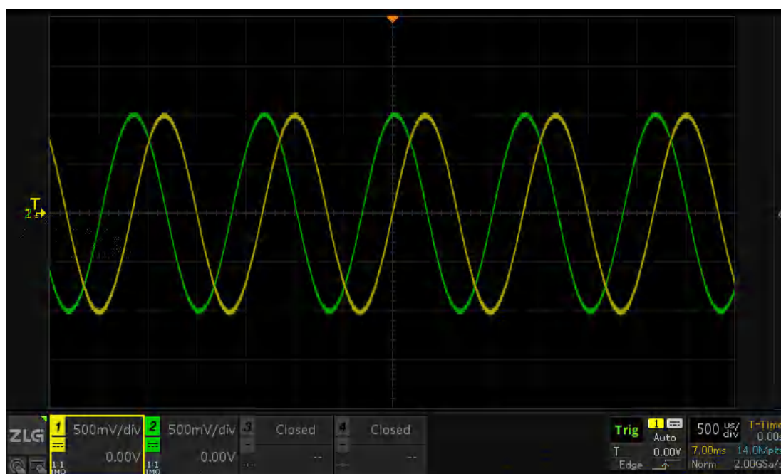
图 20.10 使能通道同步前
