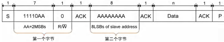
图 15.23 10 位寻址
