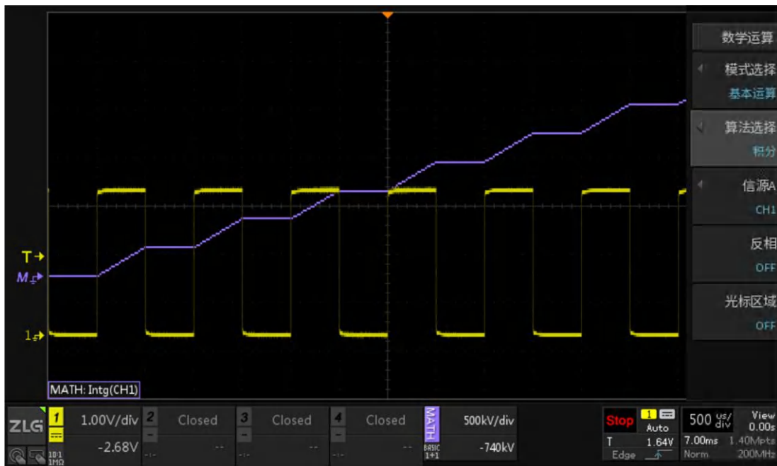
图 17.6 积分运算
