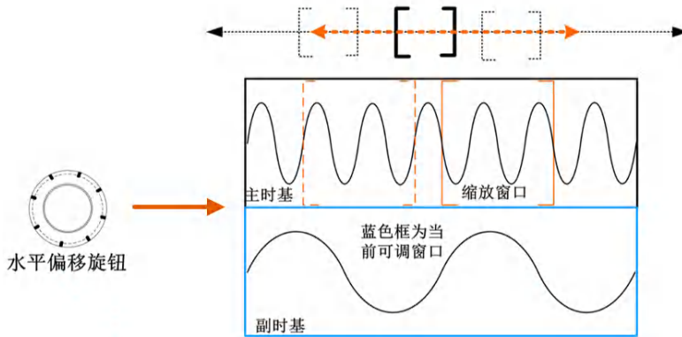
图 6.7 波形/缩放窗口偏移
