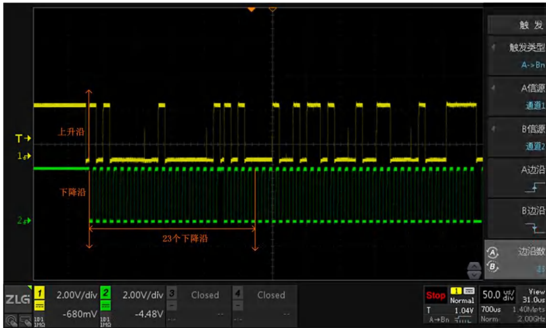
图 10.51 A-&gt;B 触发效果图
