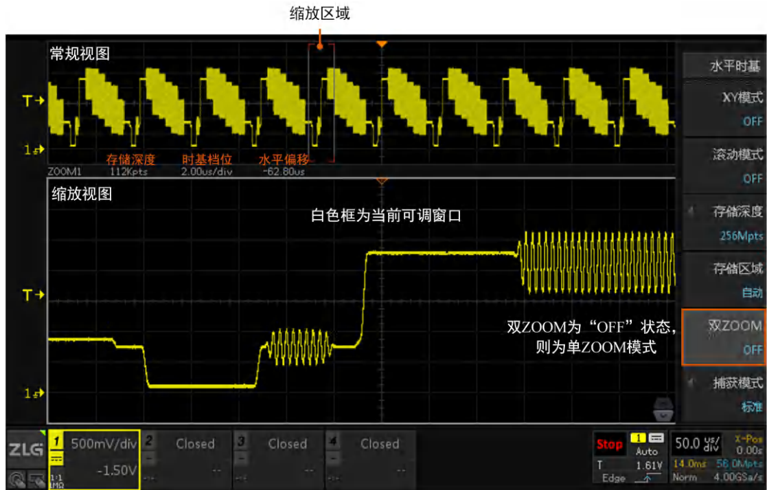
图 6.4 单 ZOOM 模式
