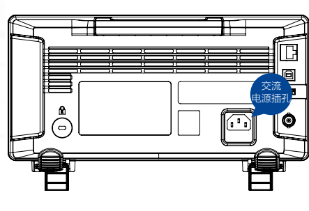
▲ 4 通道电源连接示意图
