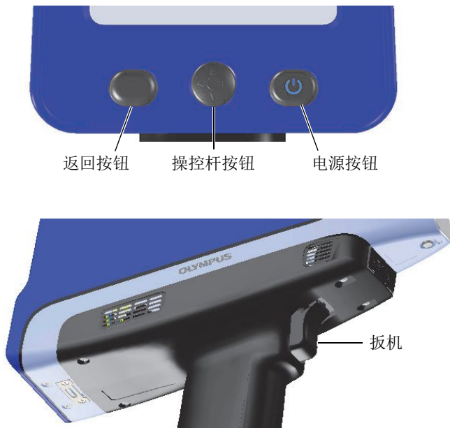
图 3-9 Vanta分析仪的外部控制装置
