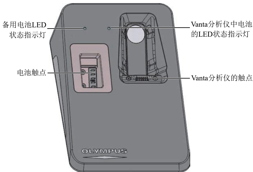
图 3-12 充电基座
