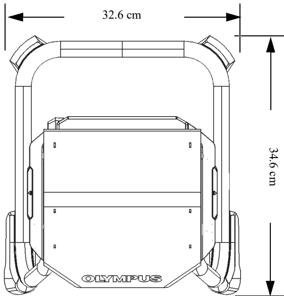
图 B-2 工作站的顶视图
