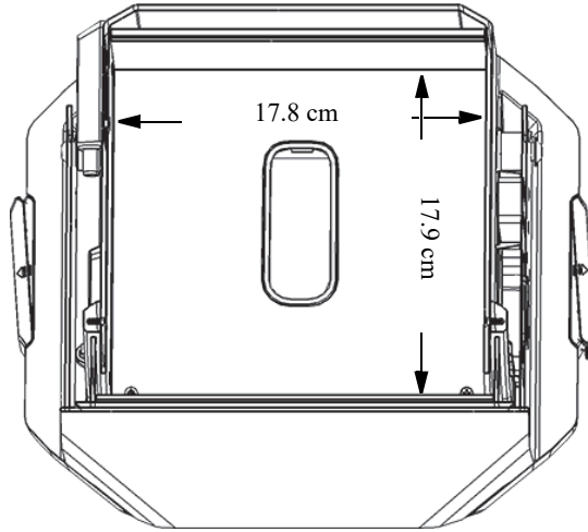
图 B-4 工作站样品舱：顶部剖面图
