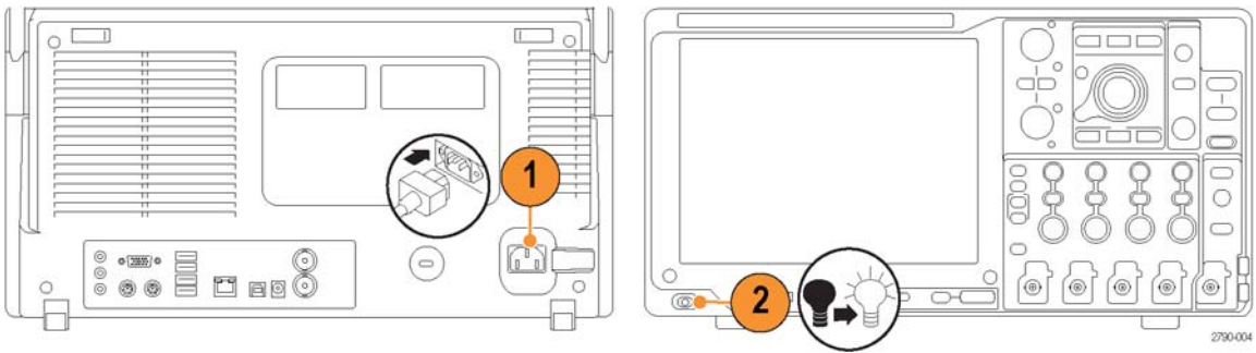
MS05000 和 DPO5000 系列
