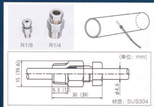
安装夹具
