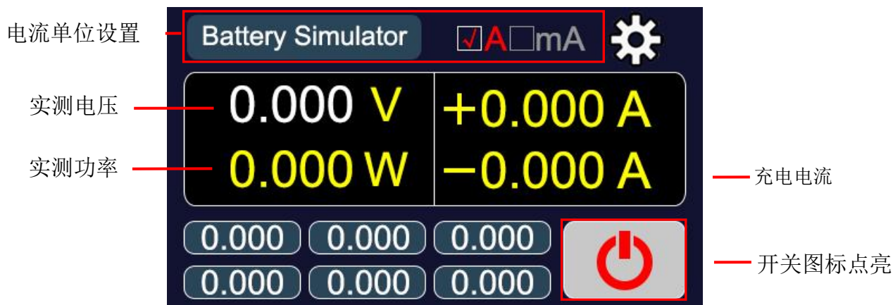
图5.4.1 可调电源
