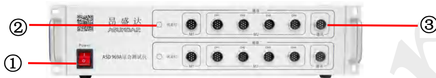
图2.2ASD969A前面板
