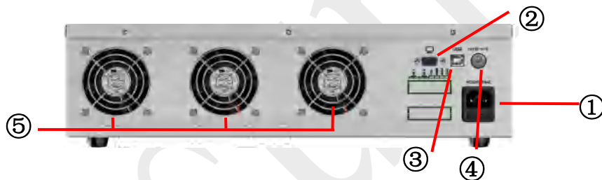
图 2.3ASD969A 后面板
