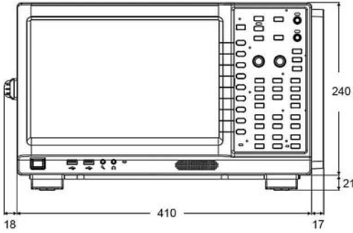
PA8000/PA6000H/PA5000H机械尺寸图 (正面)
