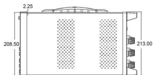
PA323/PA323H/PA333H型功率计机械尺寸图 (俯视)
