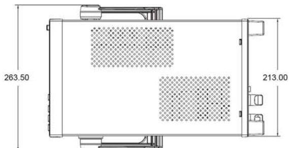
PA310型功率计机械尺寸图 (俯视)
