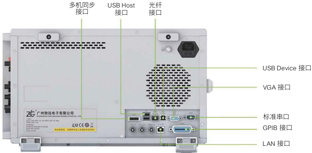
PA8000、PA5000H、PA6000H 接口图
