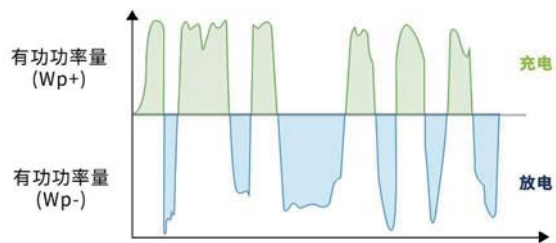
典型的重复性高速充电和放电信号
