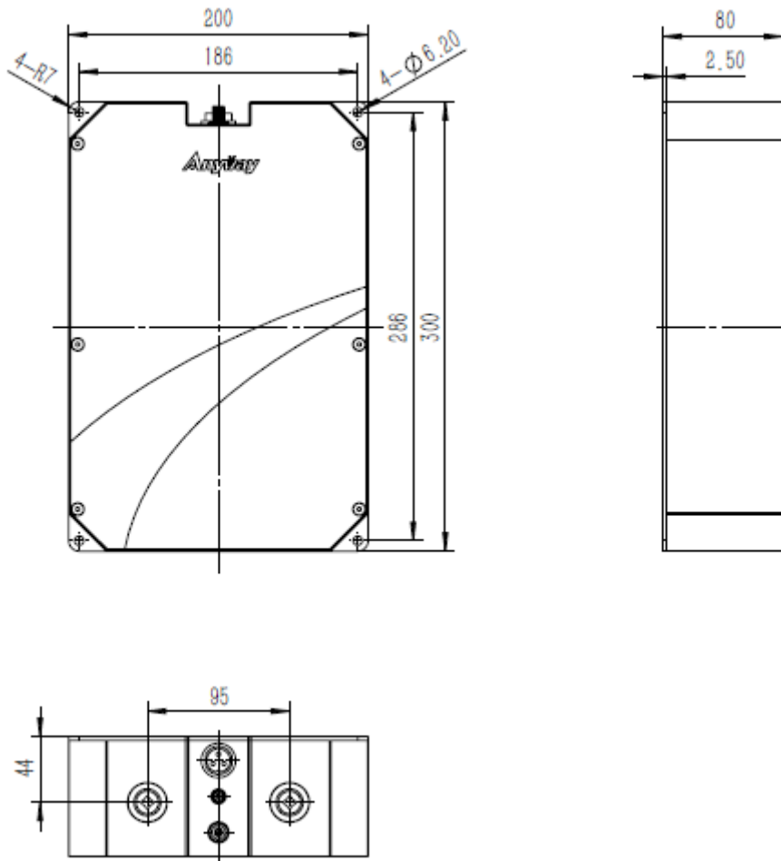
图 1 外形图
