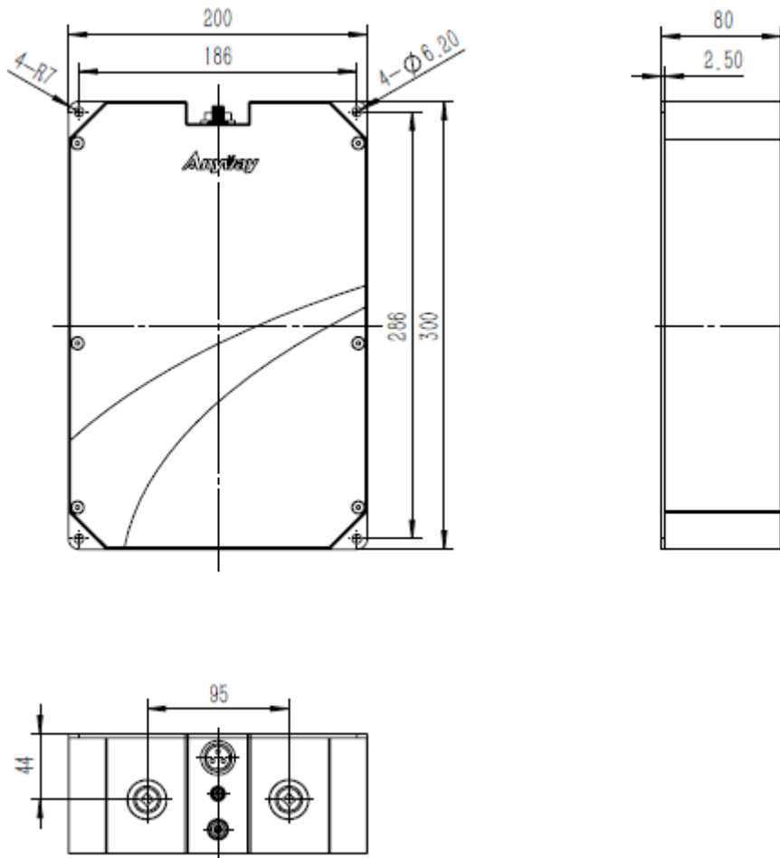
图 1 外形图
