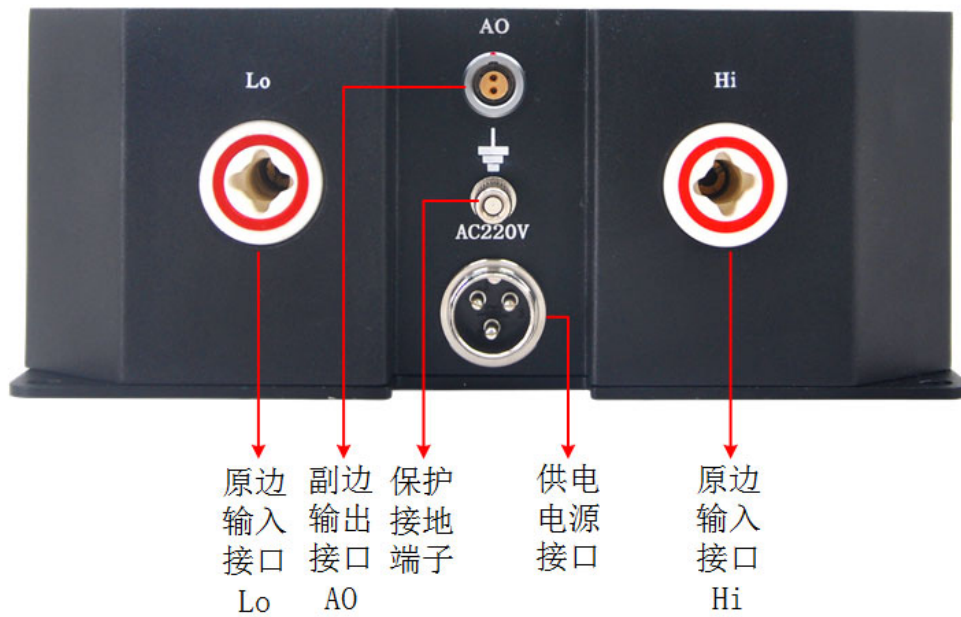
图 2 接口标识图
