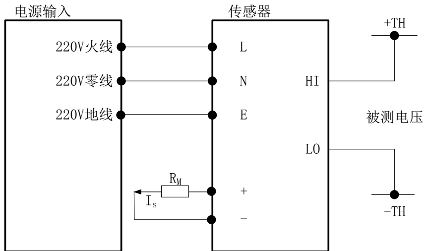
图 3 电气连接图
