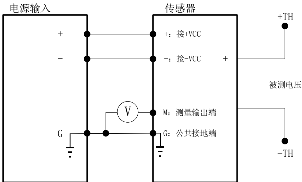
图 2 电气连接图
