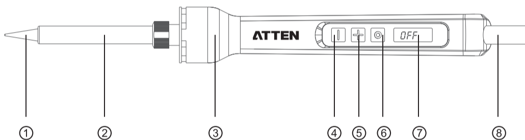
图1-1 (产品主视图)
