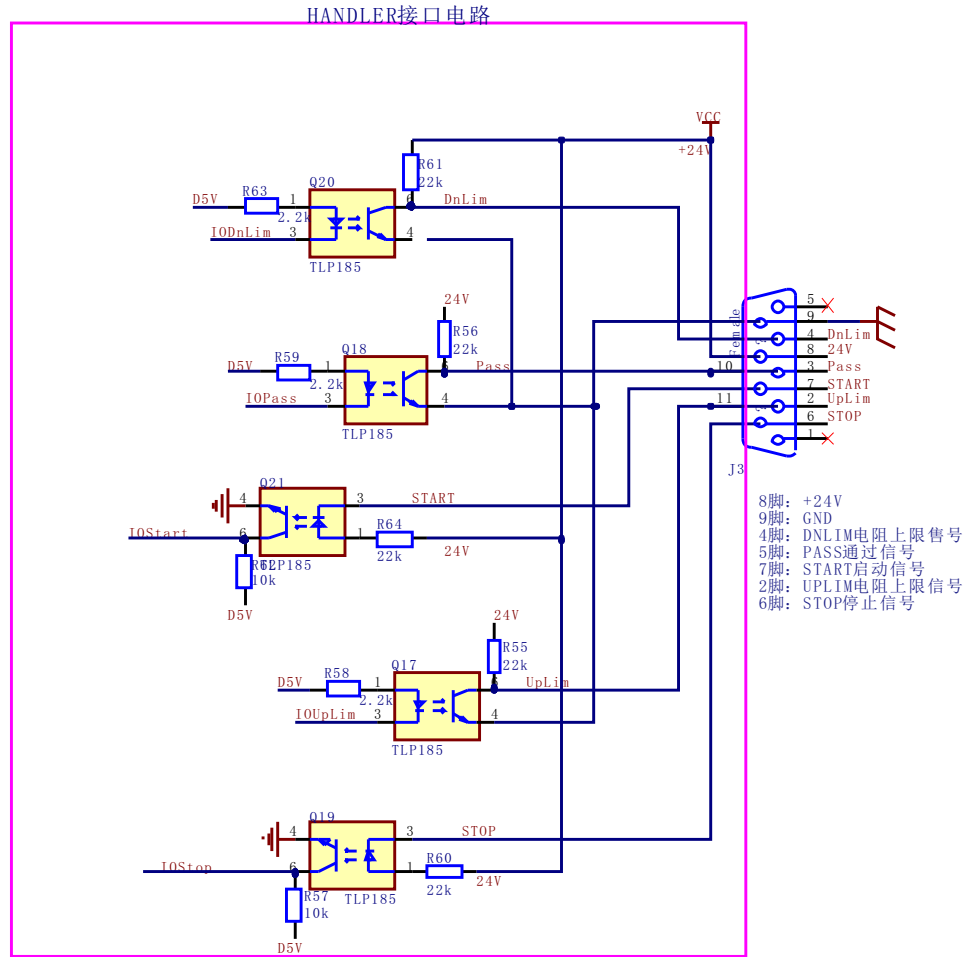
内部原理图
