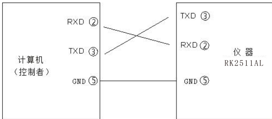
计算机与仪器接线图
