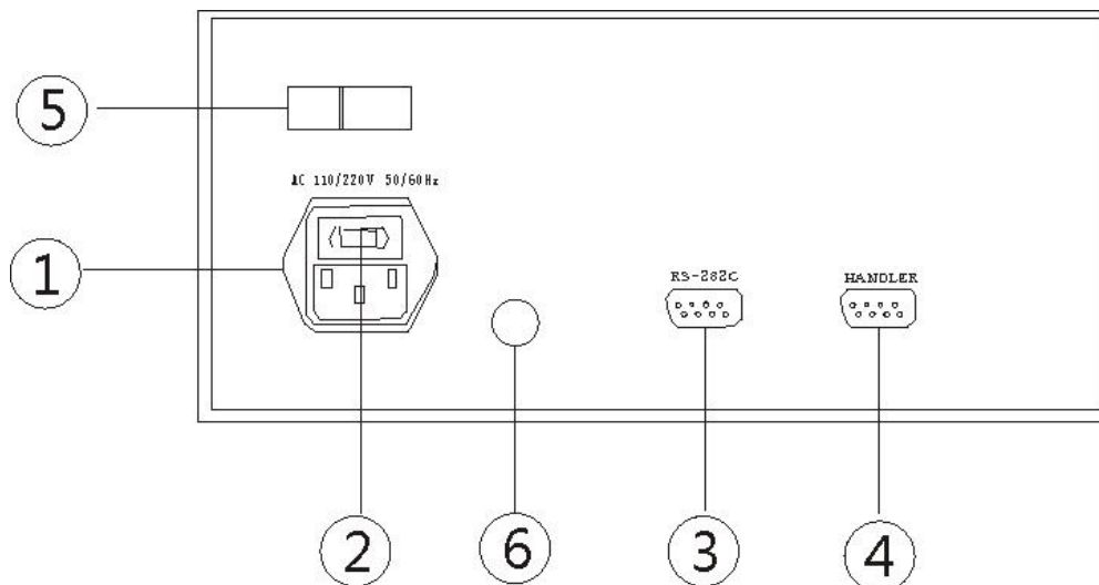
2511AL 后面板示意图
