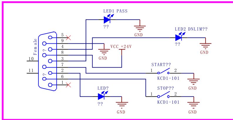
HANDLER 外部接线电路
