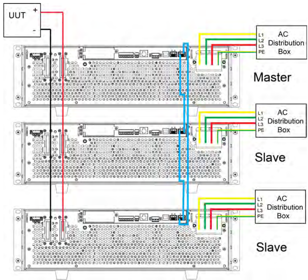
图 5-1 线路连接图
