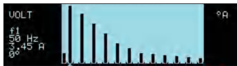
电流谐波绝对振幅条形图显示，光标位置在基波（MX30/45显示）
