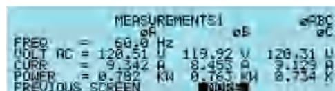
3相测量数据（MX30/45显示）
