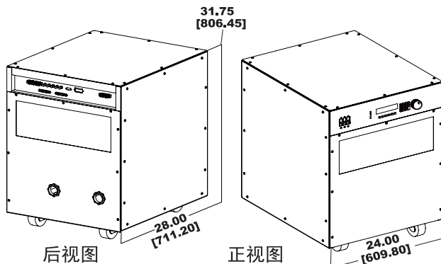
MX15 尺寸 - 单机箱
