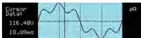
获得的电压波形（MX30/45显示）
