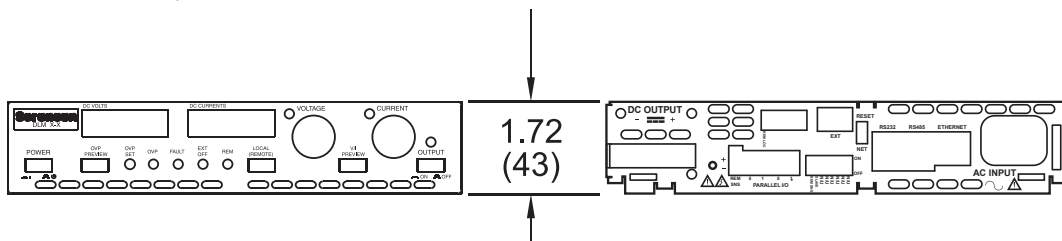
正视图
